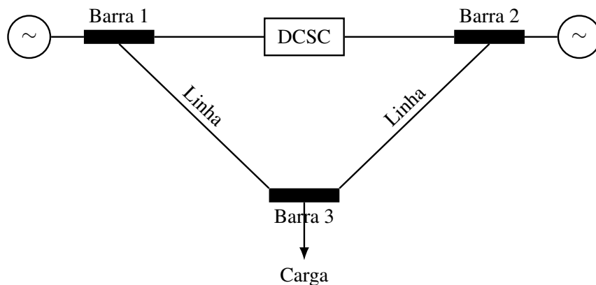
Figura 5 – Topologia da rede-exemplo 3bus_DCSC
