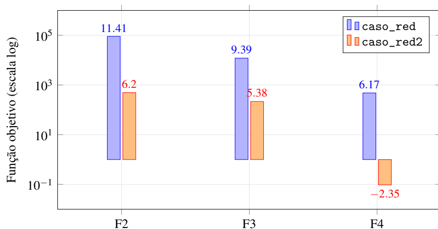
Figura 6 – Valor da função objetivo (penalização das folgas) das formulações F2, F3 e F4 sobre os casos reduzidos
