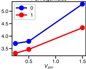
PCA eigenvalue
