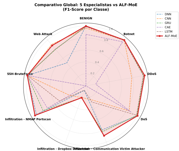
(b) CSE-CIC-IDS2018 Corrigido (L2).
