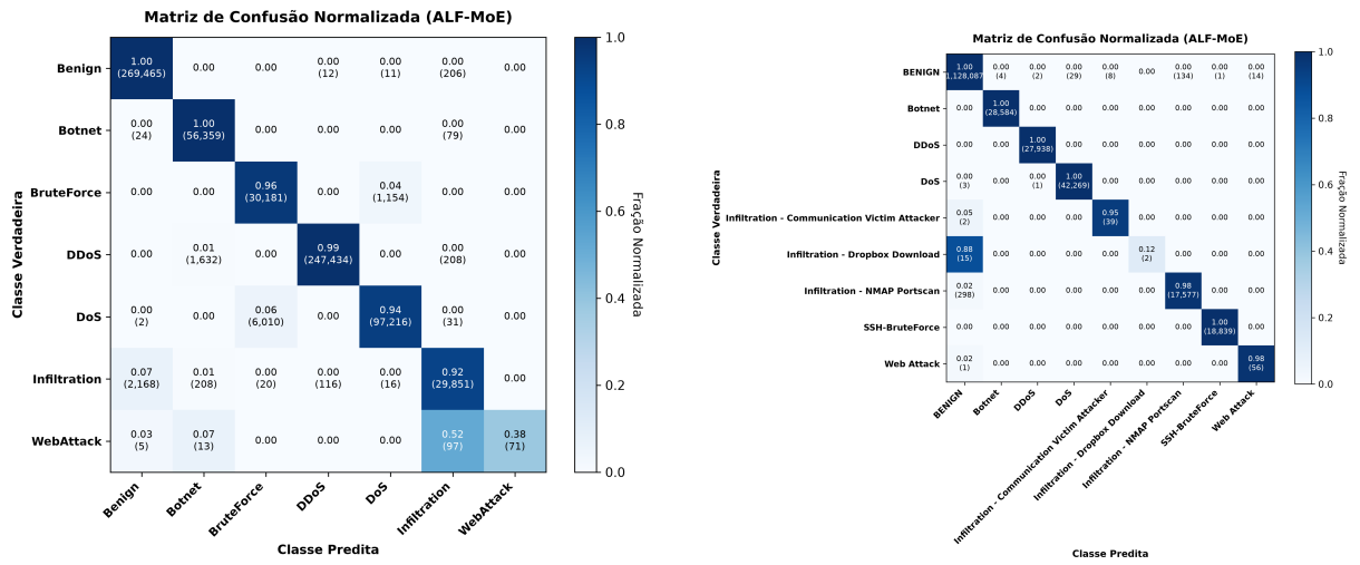
(a) CSE-CIC-IDS2018 Canônico (L2 - 7 classes).
