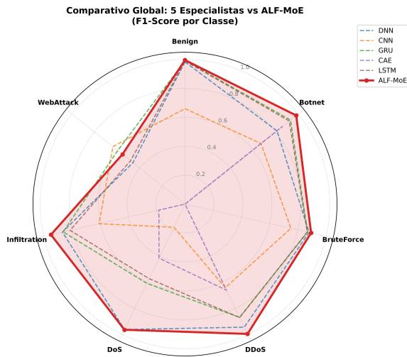
(a) CSE-CIC-IDS2018 Canônico (L2).
