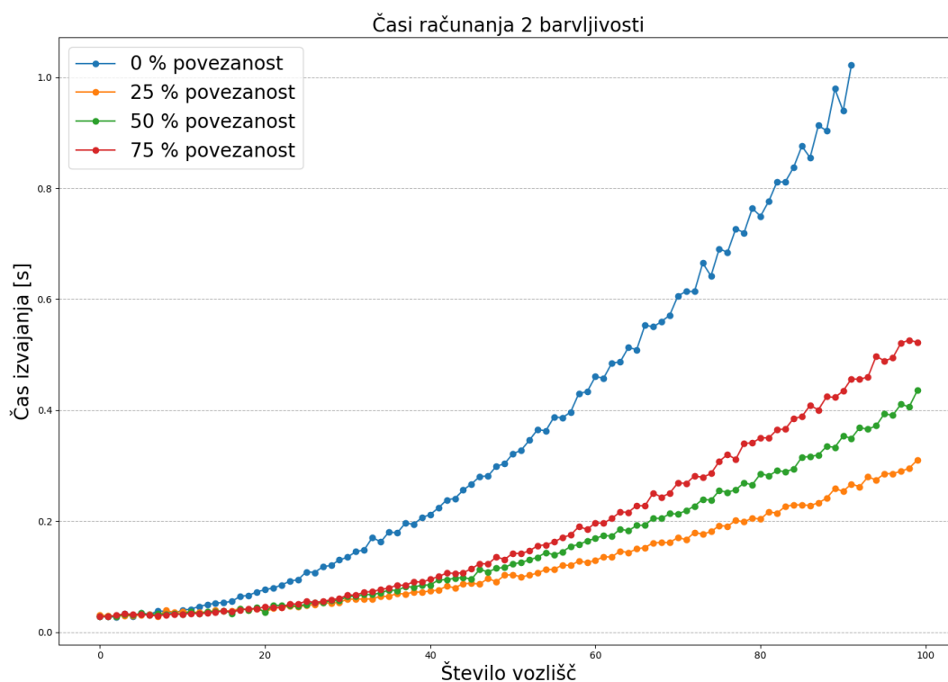
Slika 6: Poraba časa hitrega algoritma za preverjanje 2-obarvljivosti grafa G(n, p)
