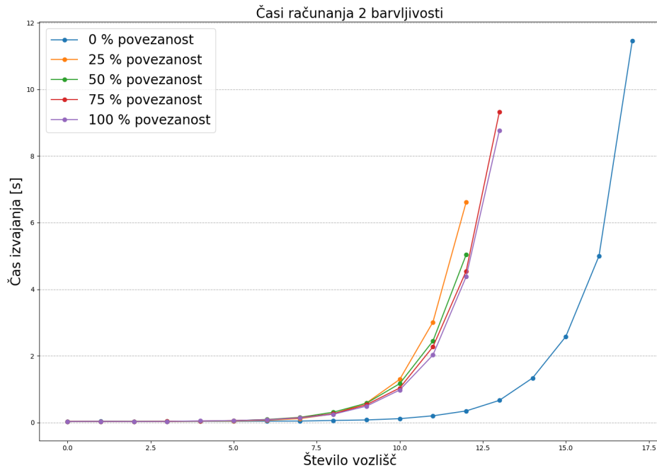
Slika 3: Poraba časa algoritma za preverjanje 2-obarvljivosti grafa G(n, p)
