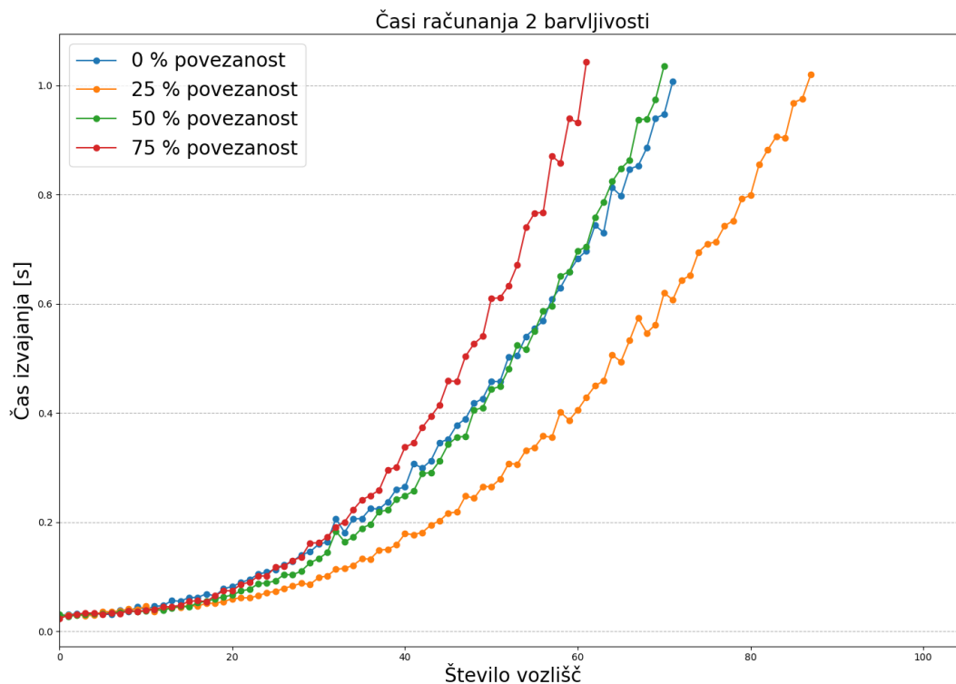
Slika 7: Poraba časa hitrega algoritma za preverjanje 2-obarvljivosti grafa G(n, p) z uporabo List
