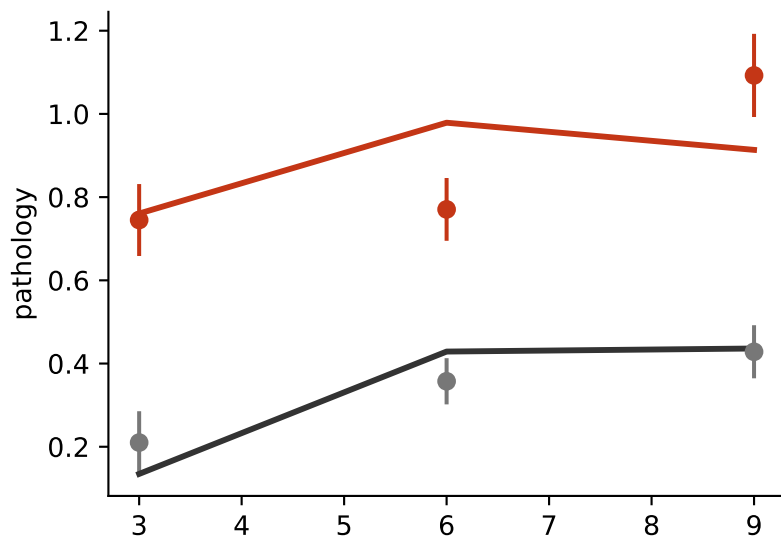
cSI: delta-PC1=2.86
