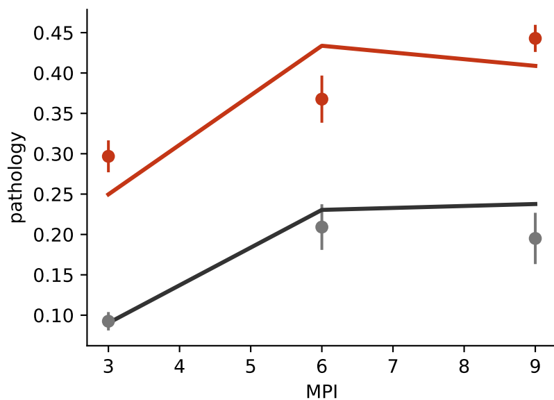
cSI: delta-PC1=2.86
