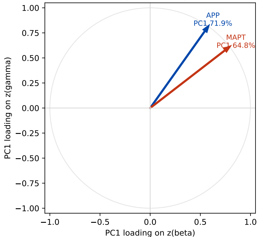
SYN PC1 directions angle=16.9 deg
