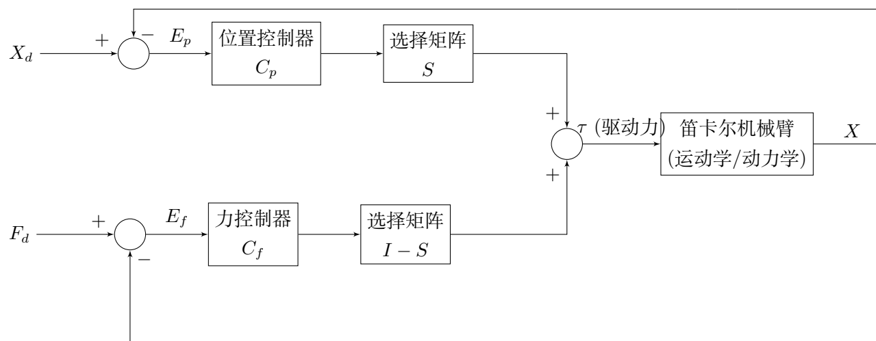
图 1: 超声波检测平台力/位混合控制系统框图 (笛卡尔空间)
