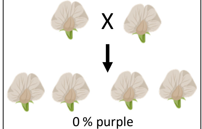
Result E
