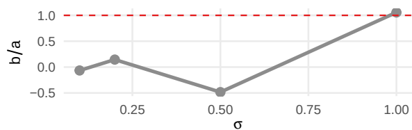
Limaçon ratio b/a
