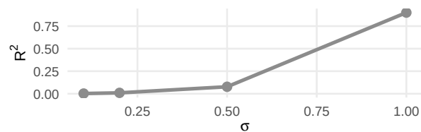
R^2 of limaçon fit
