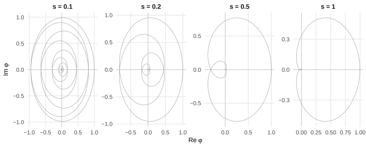
Limaçon ratio b/a
