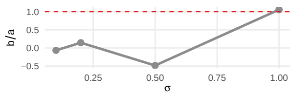
Limaçon ratio b/a
