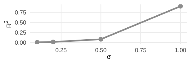
R^2 of limaçon fit
