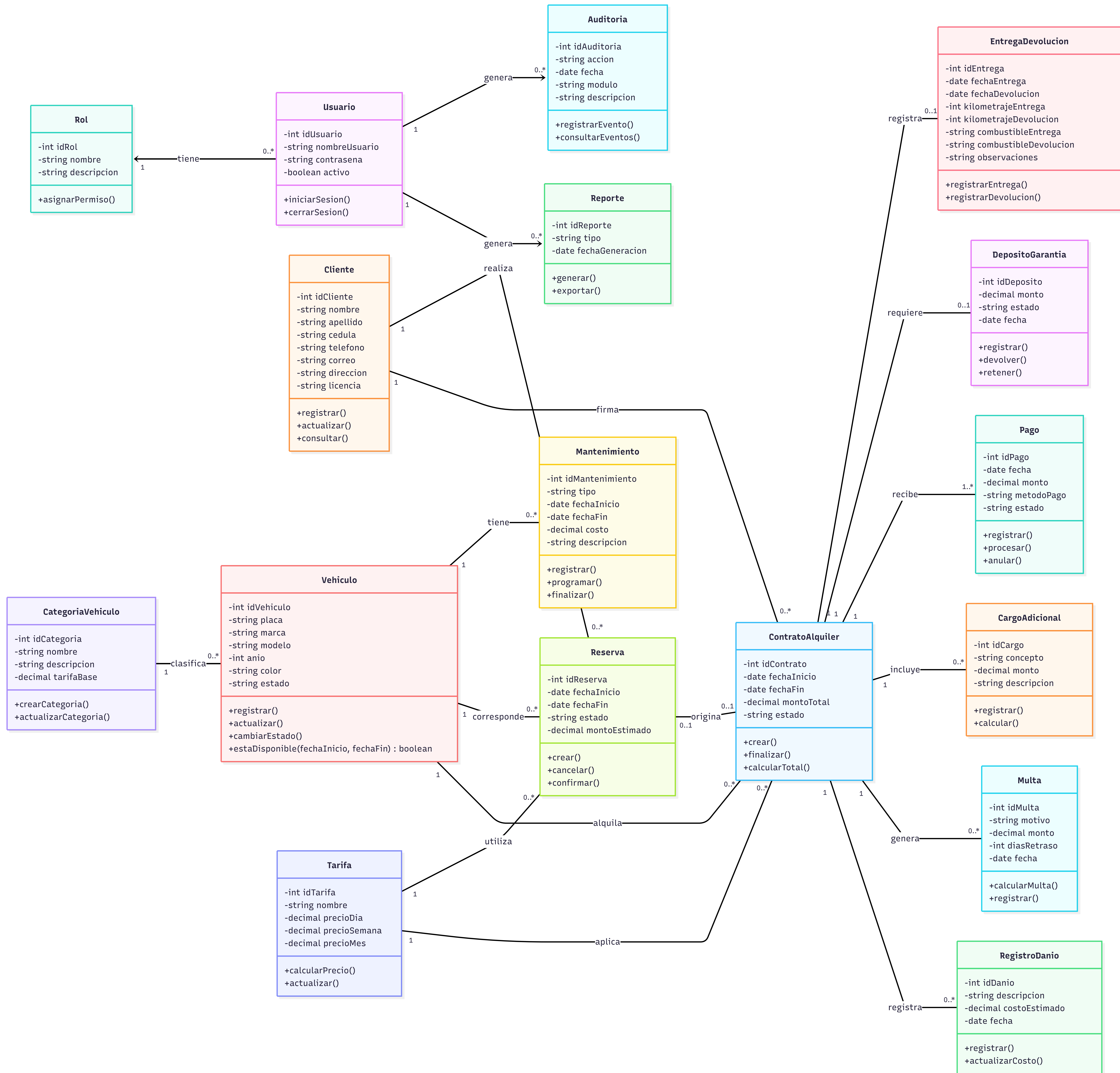
Diagrama de Clases - Sistema de Alquiler de Vehículos
