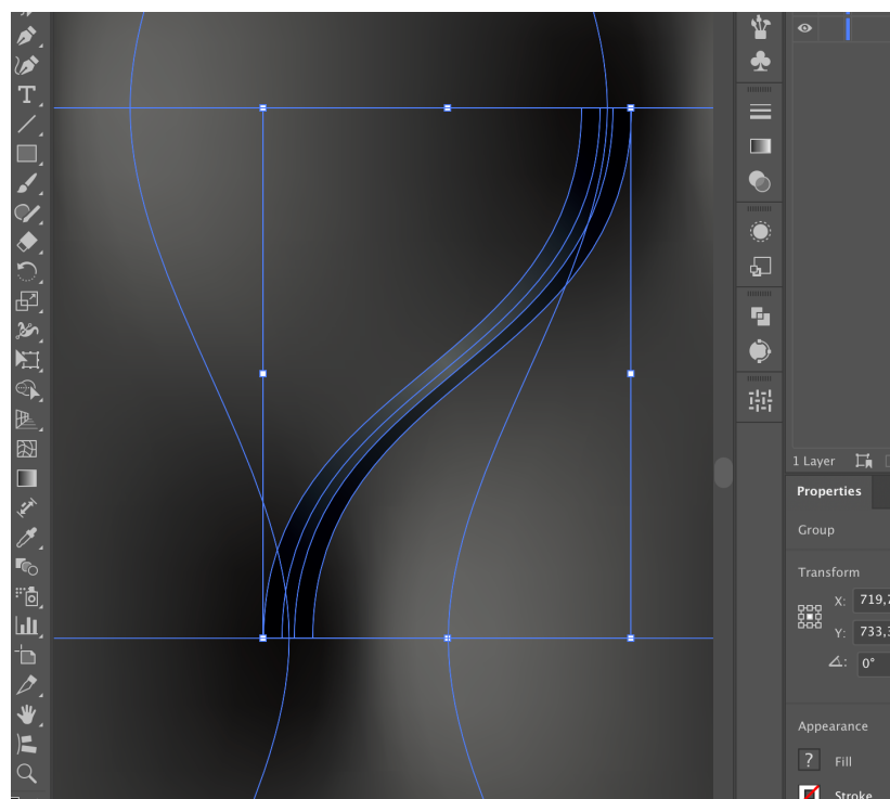
Рисунок 7 — Дублирование ленты
