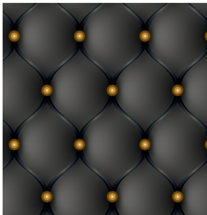
Рисунок 15 — Финальный паттерн
