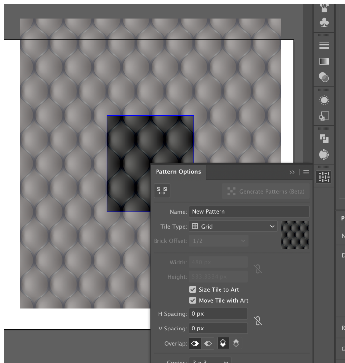
Рисунок 12 — Создание паттерна
