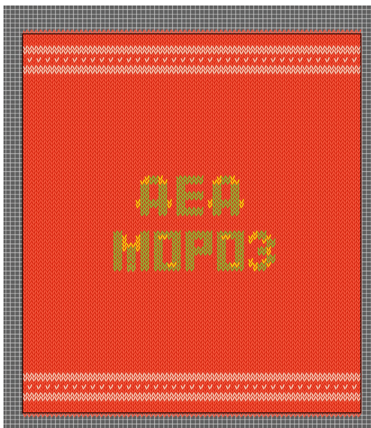
Рисунок 11 — Получившийся текст
