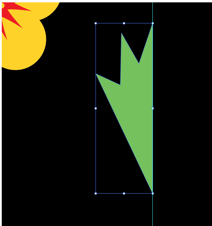
Рисунок 9 — Заготовка первой фигуры листка
