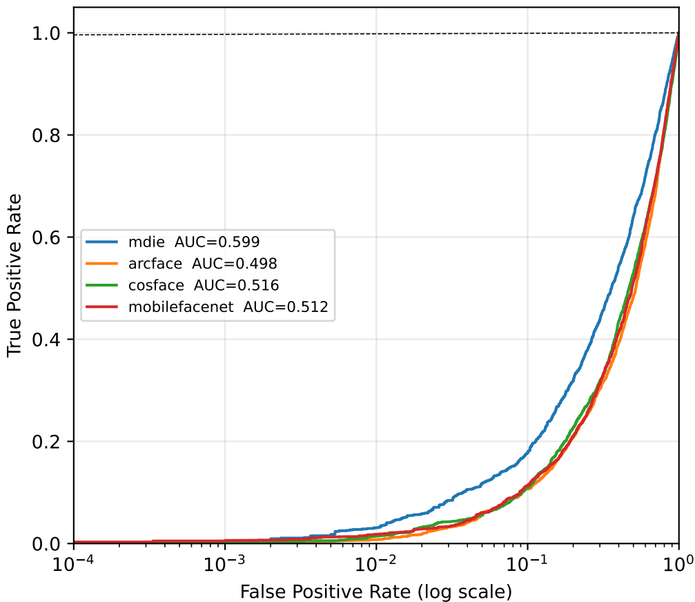
ROC — calfw
