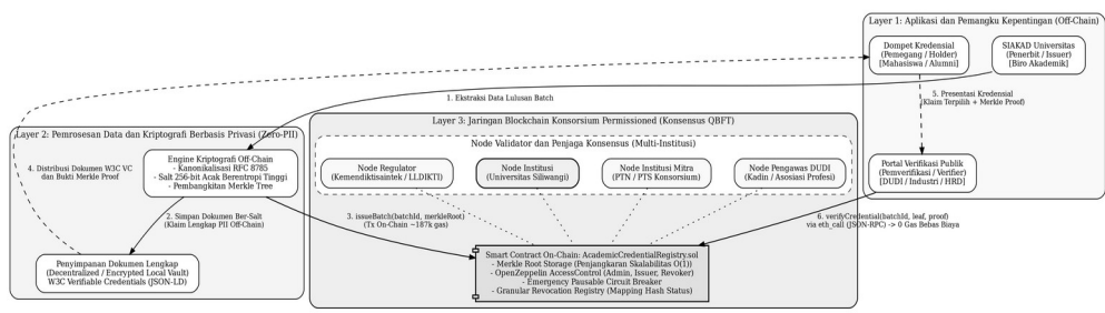
Diagram 1: Arsitektur Sistem Kredensial Akademik Konsorsium Berbasis Zero-PII dan Merkle Tree
