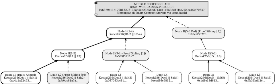
Diagram 3: Struktur Pohon Merkle Batch Wisuda dan Jalur Pembuktian (Merkle Proof Path) Daun L1
