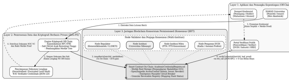
Diagram 1: Arsitektur Sistem Kredensial Akademik Konsorsium Berbasis Zero-PID dan Merkle Tree
