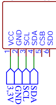
U1 BMP280
