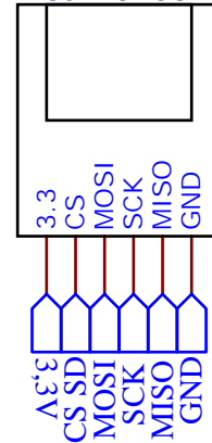
U3 MICROSD
