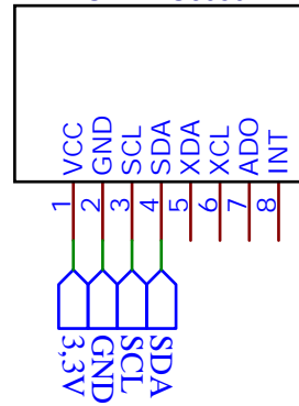
U2 MPU6050
