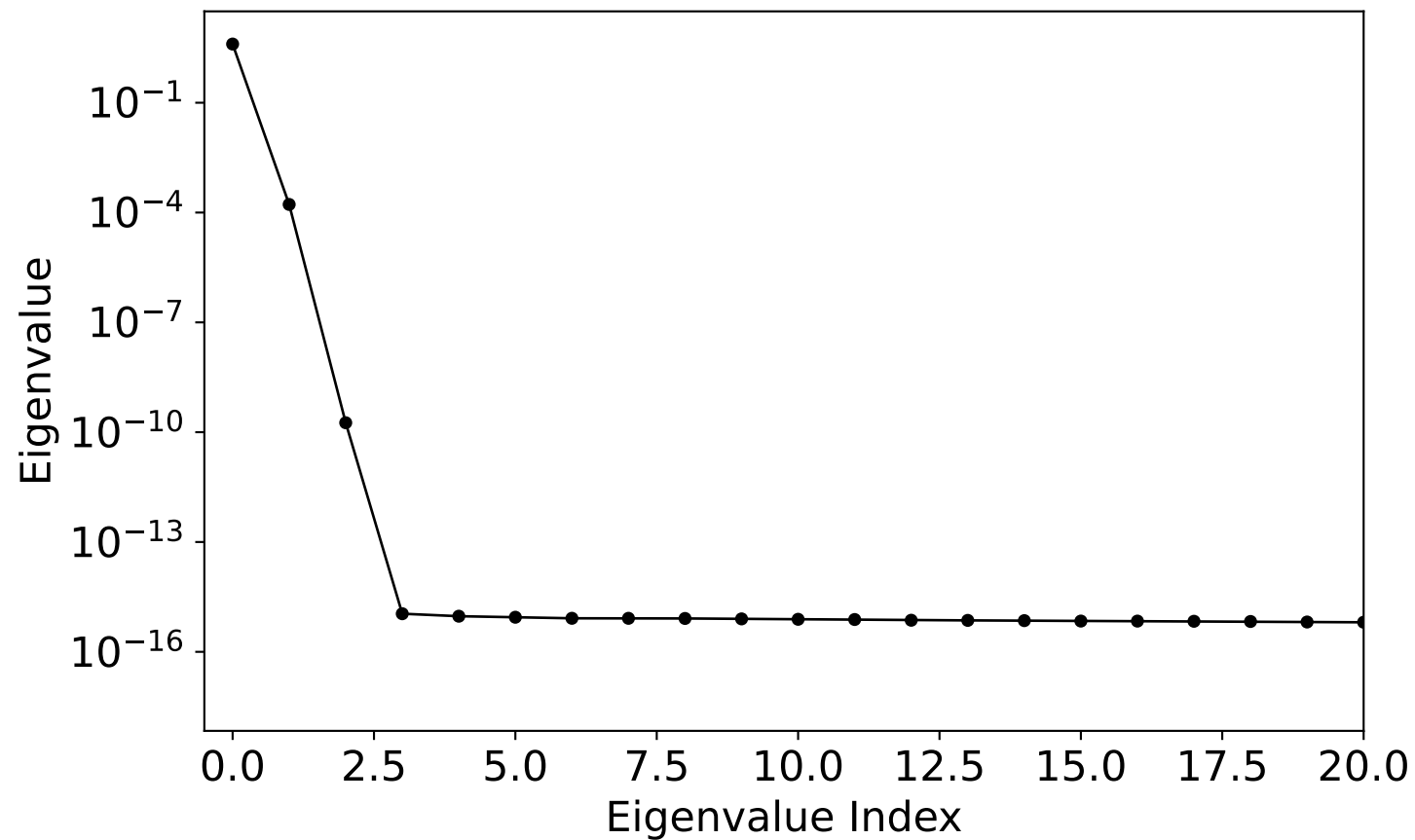
Eigenvalue vs Eigenvalue Index
