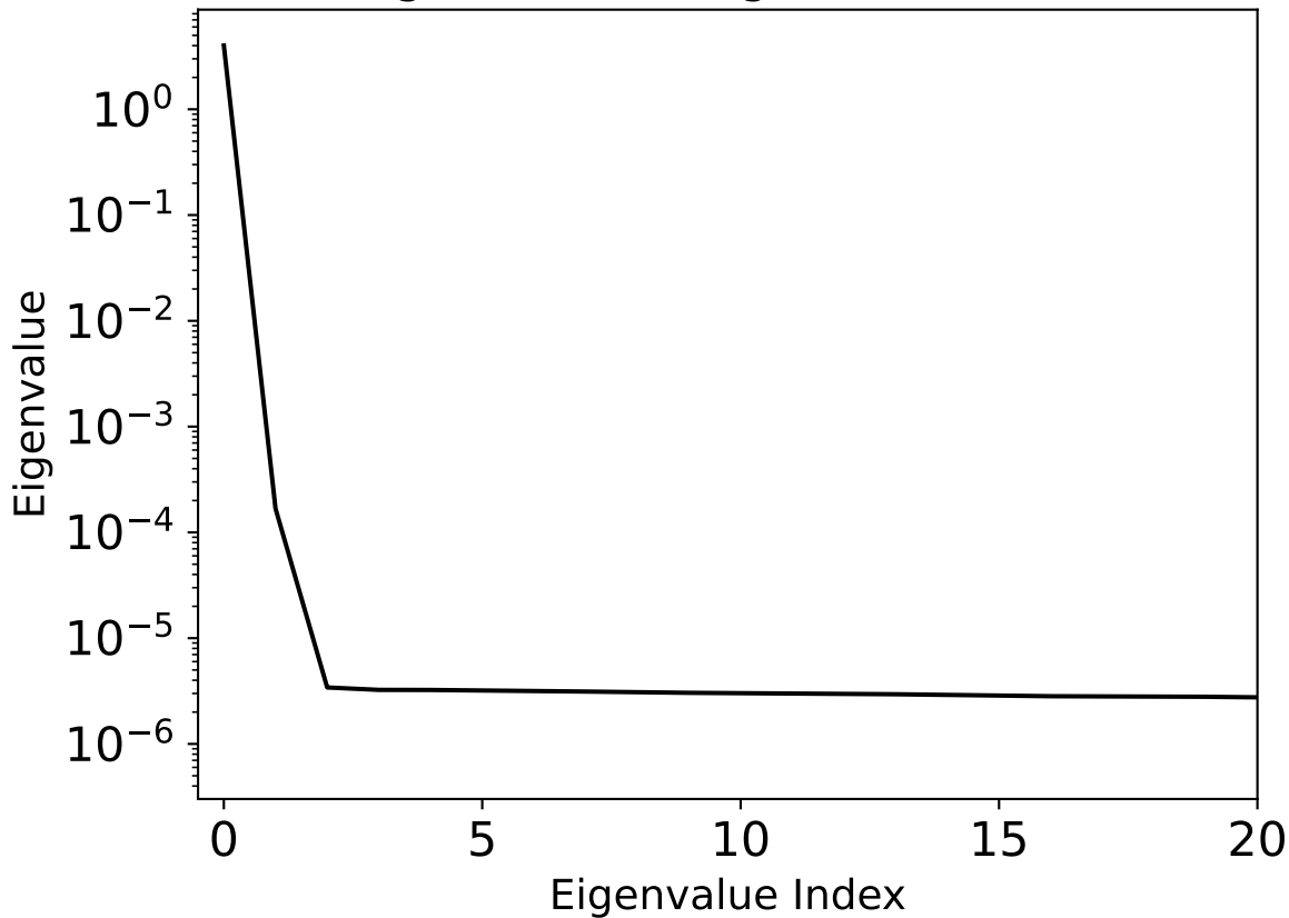
Eigenvalue vs Eigenvalue Index
