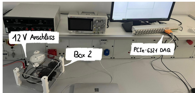
Abbildung 4: Setup des Versuchs.
