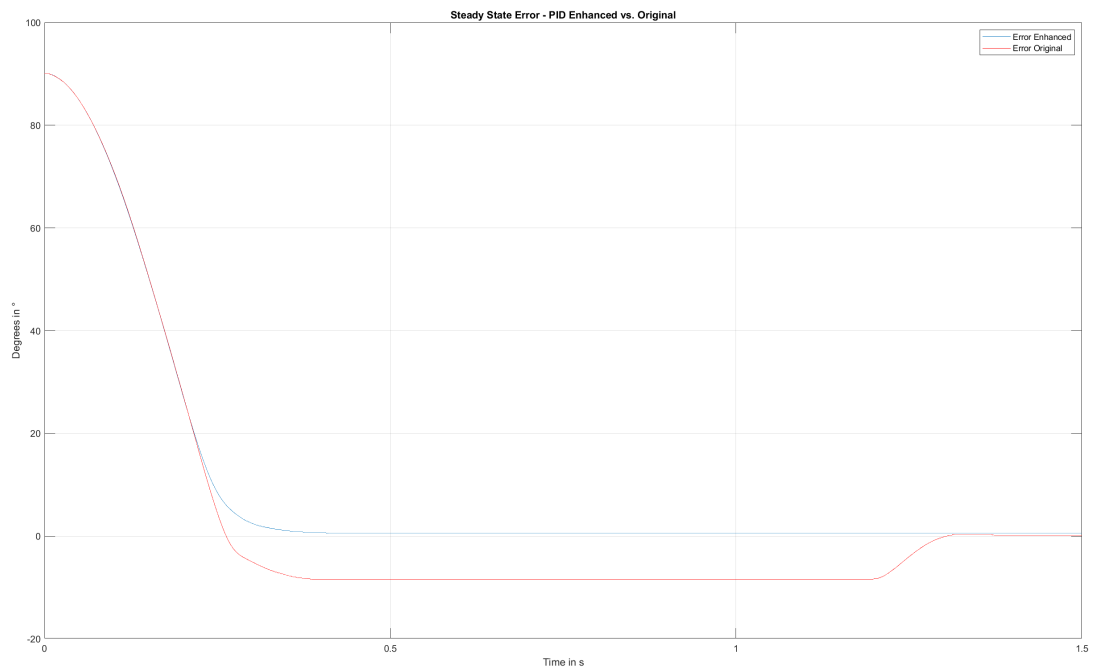
Abbildung 10: Steady-State-Error-Vergleich der Systeme mit verschiedenen Koeffizienten. Die XXX Funktion beinhaltet die berechneten Werte für den PID-Controller und die XXX Funktion die angepassten Werte.
