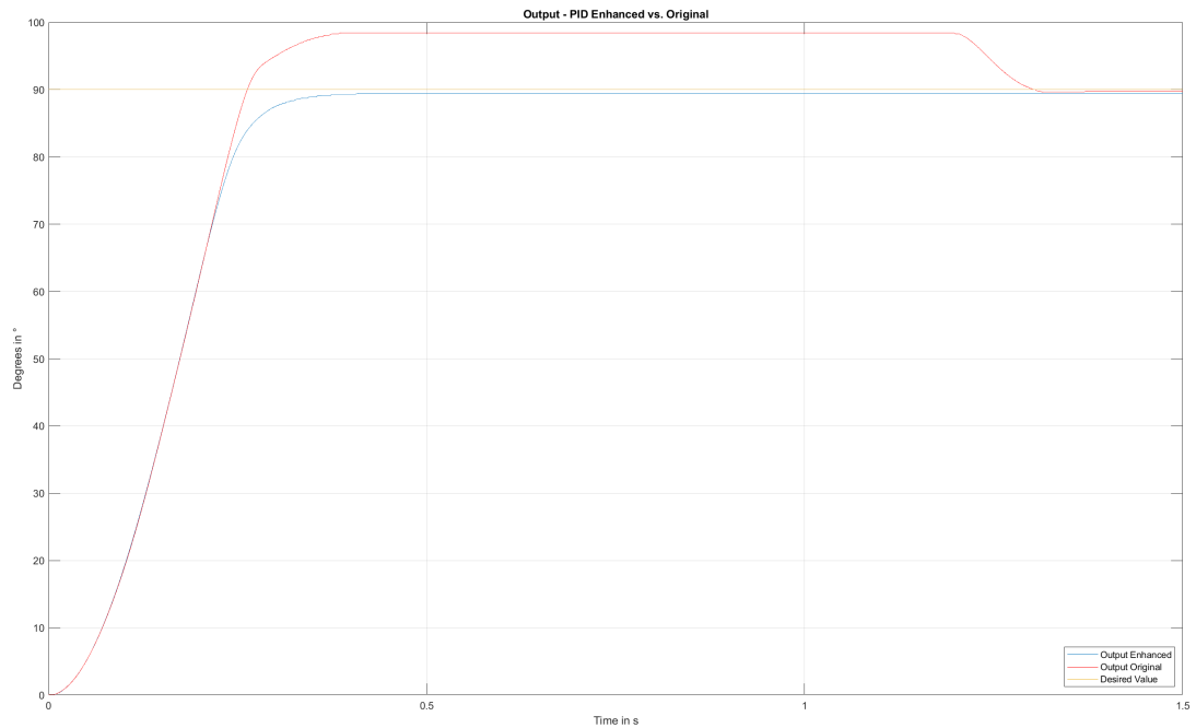
Abbildung 9: Output-Vergleich der Systeme mit verschiedenen Koeffizienten. Die XXX Funktion beinhaltet die berechneten Werte für den PID-Controller und die XXX Funktion die angepassten Werte.
