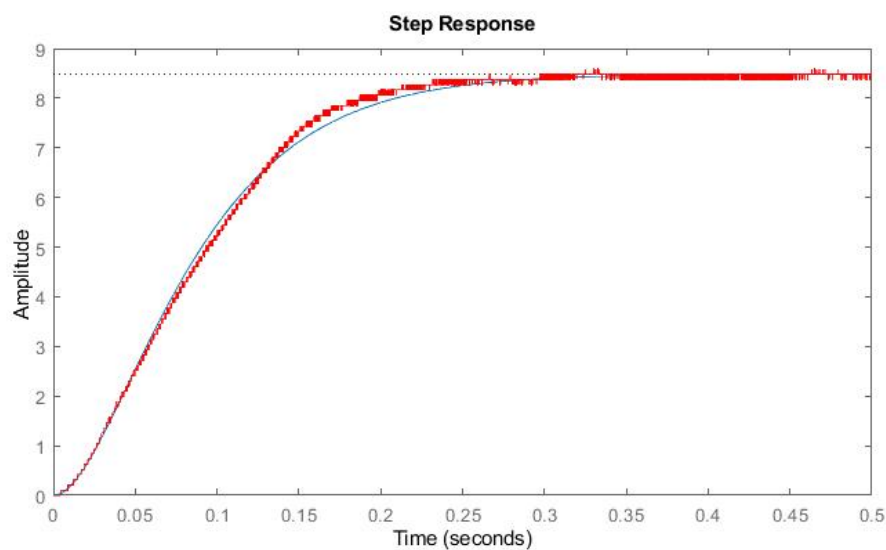
Abbildung 4: Step Response des Systems. Eine Gegenüberstellung der gemessenen Daten und der berechneten Übertragungsfunktion zeigen eine S-Kurve.
