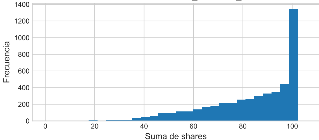
Distribución de share_1 + share_2
