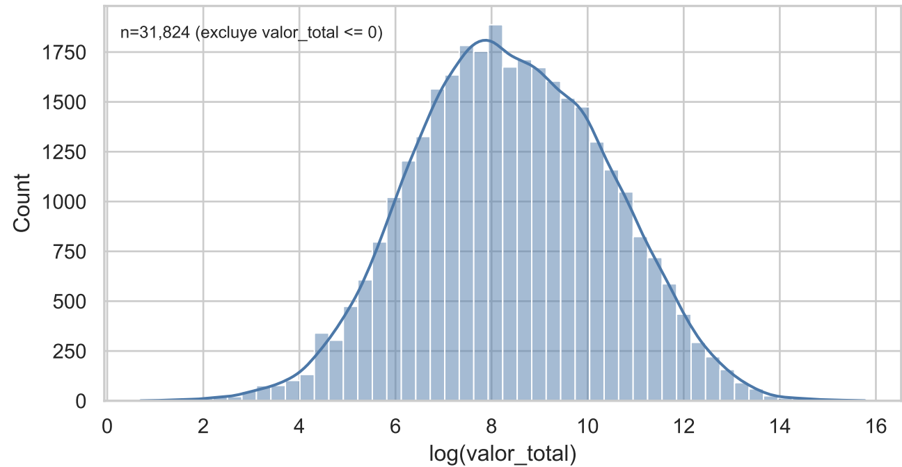
Log(valor_total) (solo valores positivos)
