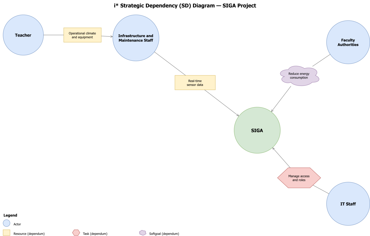
Figura 8: Modelo i* de Dependencia Estratégica (SD) del proyecto SIGA
