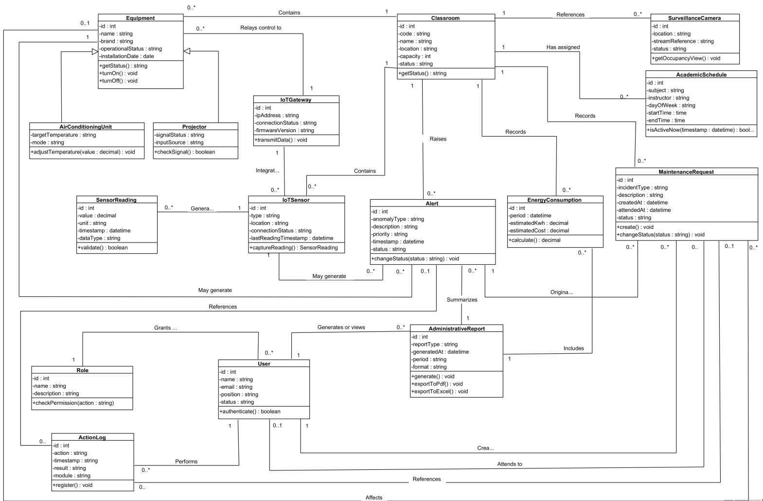
Figura 5: Modelo de clases refinado del dominio de SIGA
