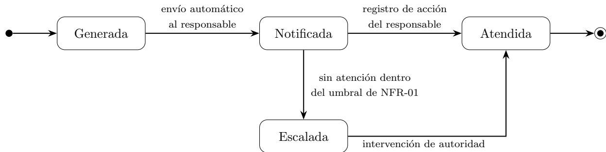
Figura 6: Diagrama de estados de la entidad Alerta , redibujado conforme a la §4.6 del ERS (defecto D-15)
