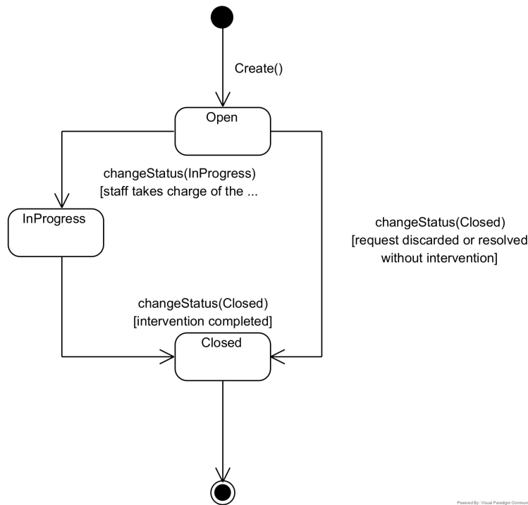
Figura 7: Diagrama de estados de la entidad SolicitudMantenimiento
