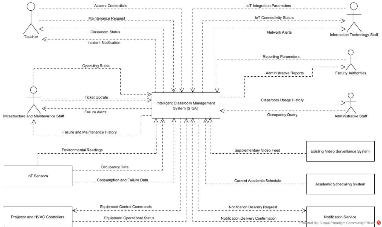
Figura 2: Diagrama de contexto del sistema SIGA
