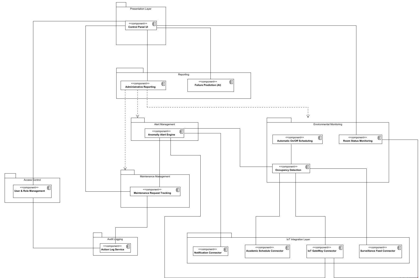
Figura 3: Diagrama de componentes del sistema SIGA
