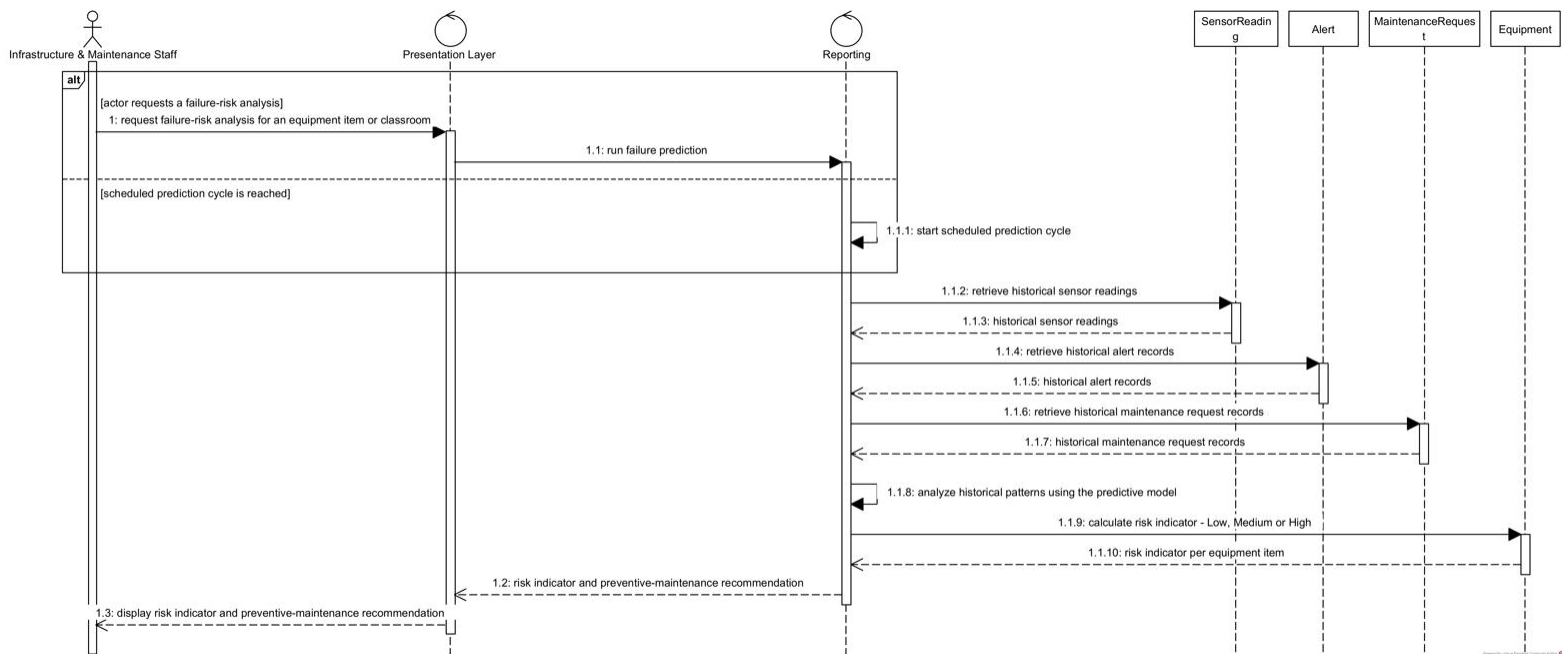
Figura 10: Diagrama de secuencia de CU-16, predicción de fallas de equipos
