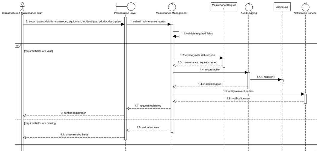
Figure 24: Diagrama de secuencia — CU-06 Registrar solicitud de mantenimiento
