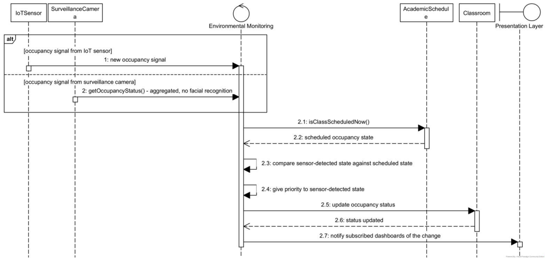
Figure 21: Diagrama de secuencia — CU-03 Detectar ocupación de aula
