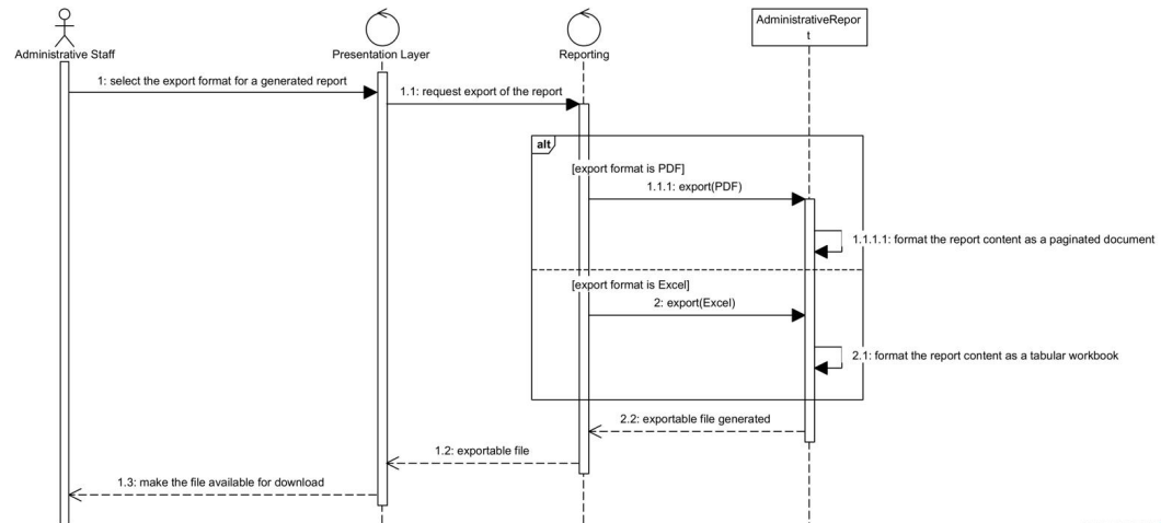
Figure 28: Diagrama de secuencia — CU-10 Exportar reportes PDF y Excel
