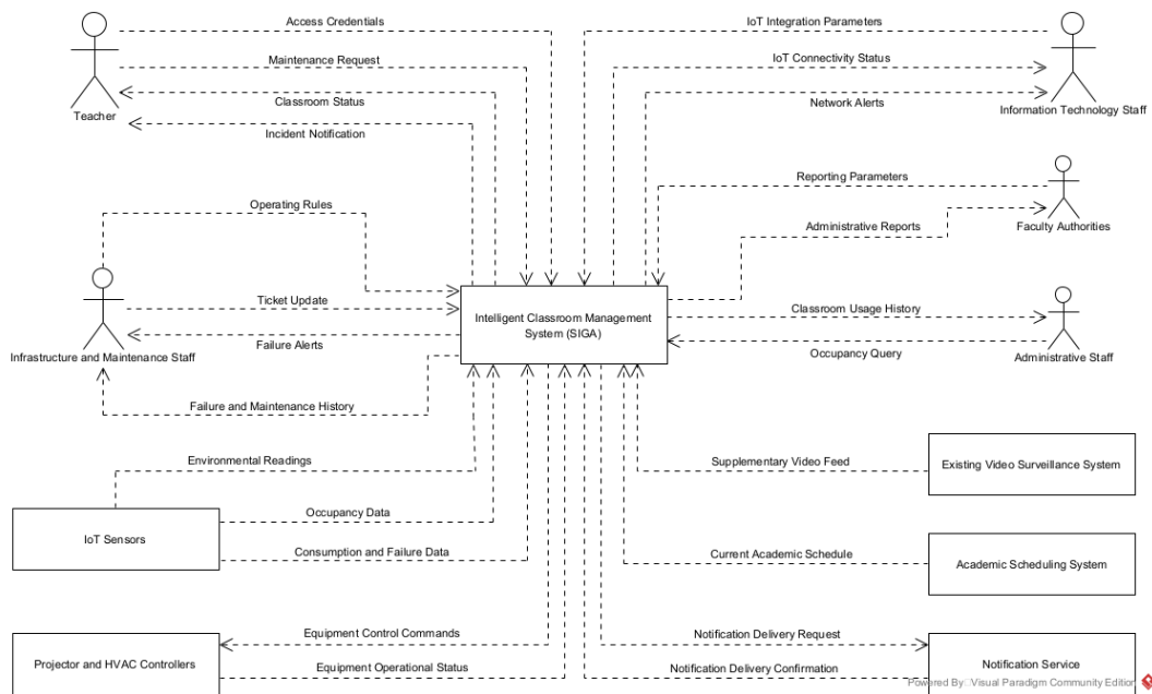
Figure 2: Diagrama de contexto
