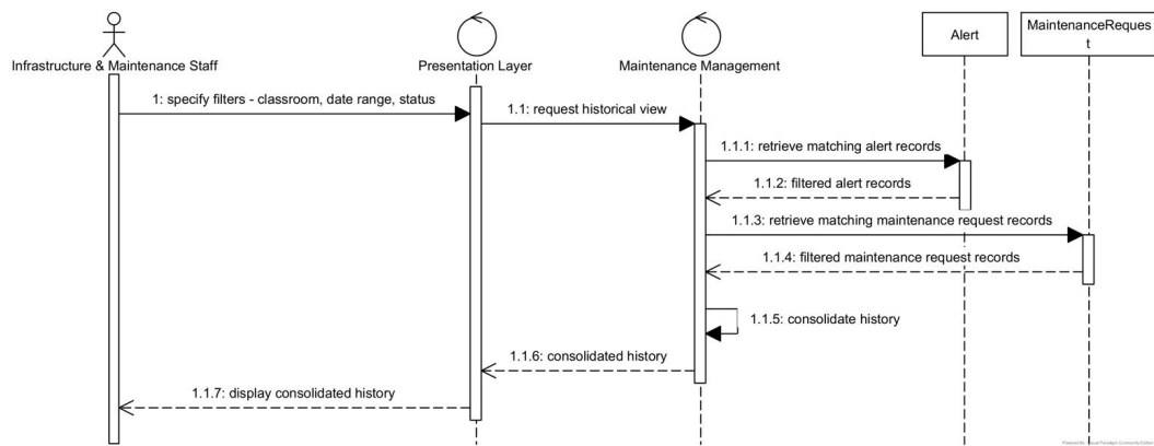
Figure 26: Diagrama de secuencia — CU-08 Consultar historial de fallas y mantenimientos
