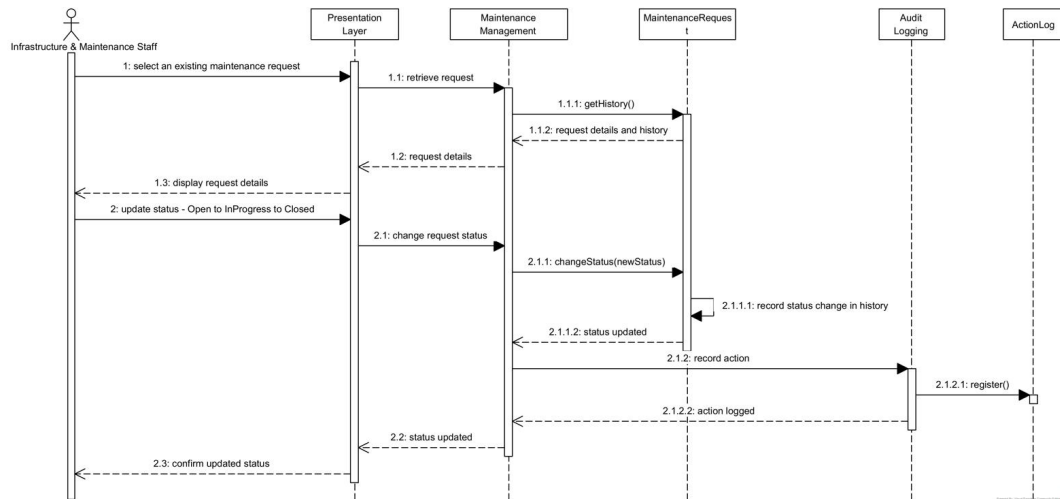
Figure 25: Diagrama de secuencia — CU-07 Dar seguimiento a ticket de mantenimiento
