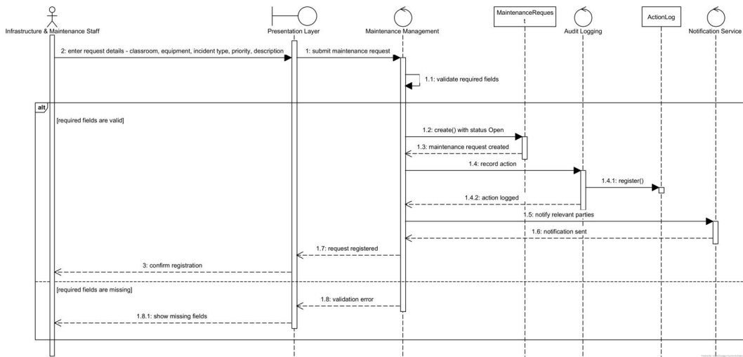
Figure 12: Diagrama de secuencia — CU-06 Registrar solicitud de mantenimiento
