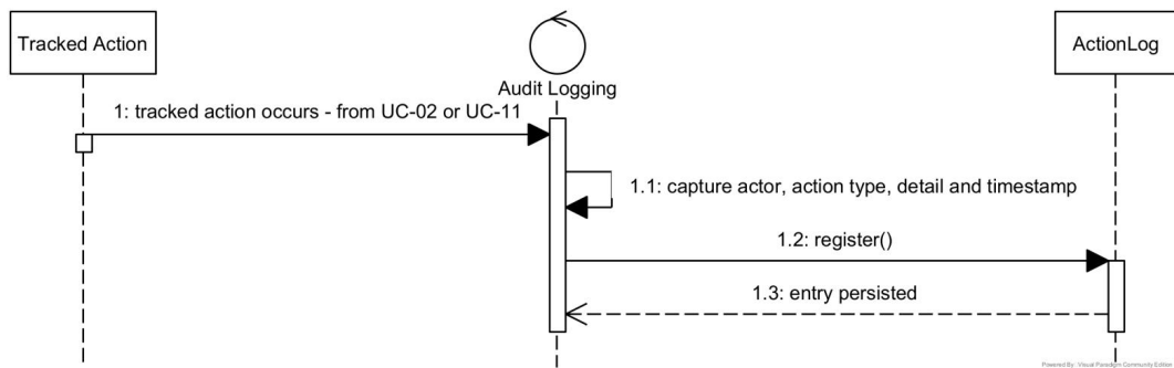
Figure 32: Diagrama de secuencia — CU-14 Registrar bitácora de acciones
