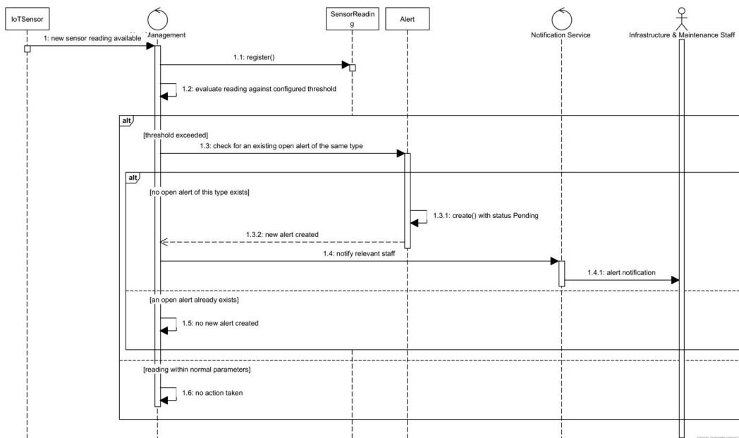
Figure 22: Diagrama de secuencia — CU-04 Generar alertas por anomalías
