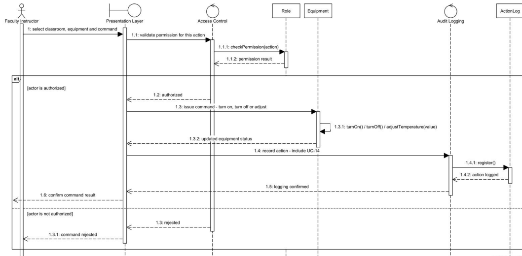
Figure 20: Diagrama de secuencia — CU-02 Controlar remotamente equipos de aula
