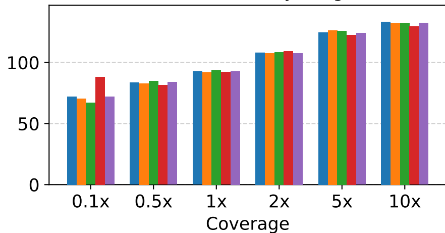
(D) MIQP Memory Usage
