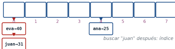
Figura 7.5: Encadenamiento paso a paso: "juan" entra en el balde 0 y "ana" en el 4 sin conflicto; cuando "eva" también da 0, simplemente se encadena en ese balde. Buscar recorre sólo la cadena de su balde.
