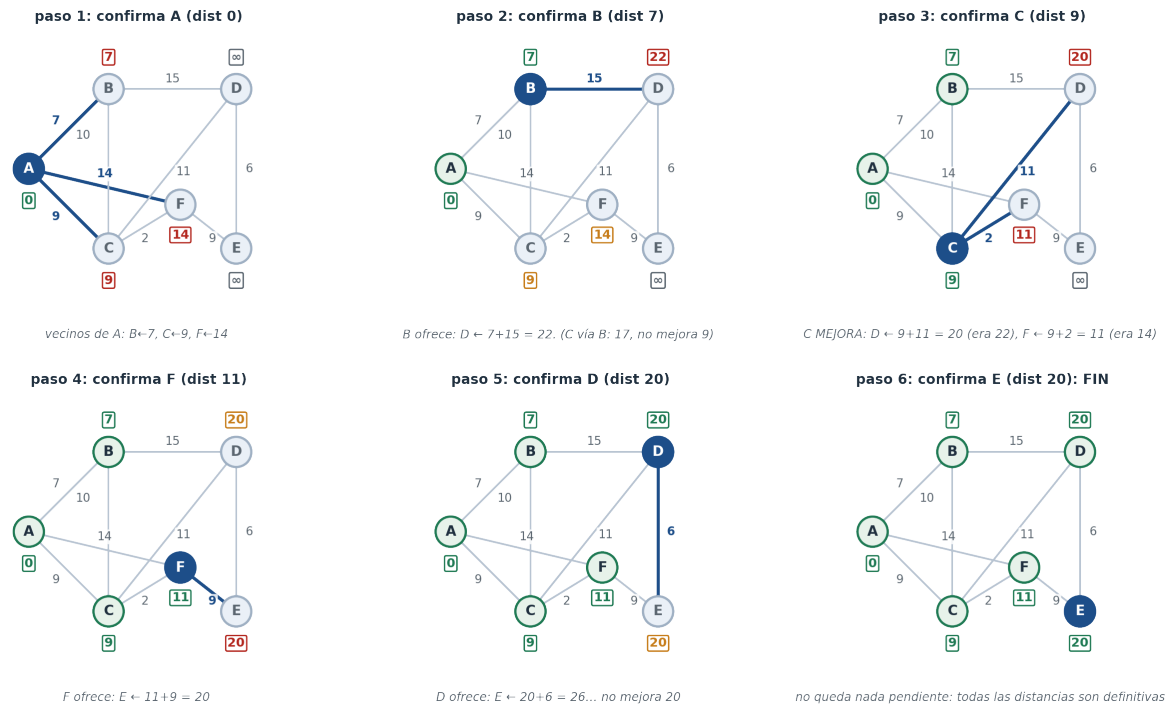
Figura 11.7: Dijkstra paso a paso desde A. Cada panel confirma un vértice (azul), que pasa a verde con su distancia definitiva. Los recuadros muestran la mejor distancia conocida: rojo = recién actualizada, naranja = pendiente, verde = confirmada. Mirá el paso 3: C mejora a D (22 → 20) y a F (14 → 11) — el camino directo A–F nunca fue la respuesta.
