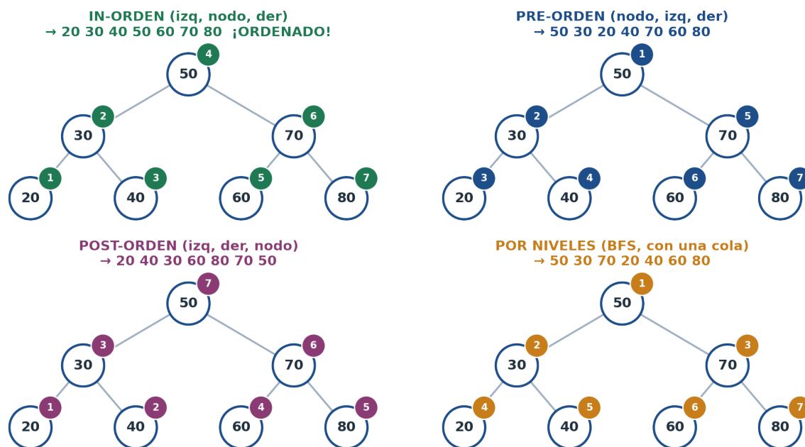
Figura 8.6: Los cuatro recorridos sobre el mismo árbol, con el orden de visita numerado en cada nodo. El in-orden de un ABB entrega los valores ordenados.
