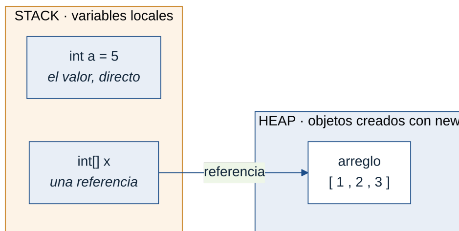
Figura 2.1: Los primitivos locales viven en el stack; los objetos, en el heap. Una variable de objeto guarda una referencia al heap.
