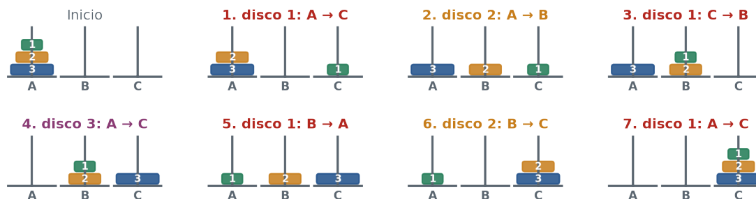
Figura 6.11: Torres de Hanói con 3 discos: los 7 movimientos, uno por panel. Movimientos 1-3: la torre de 2 discos se corre a B (destrabando el disco 3). Movimiento 4: el disco grande viaja a C. Movimientos 5-7: la torre de 2 se rearma encima.
