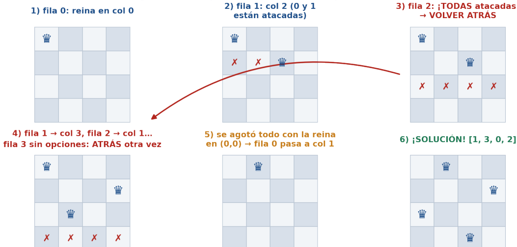
Figura 10.2: Las 4 reinas paso a paso: se avanza fila por fila; cuando la fila 2 se queda sin columnas válidas, se vuelve atrás y se mueve la reina anterior. Tras agotar todo lo que empezaba en (0,0), la primera reina se corre — y aparece la solución [1, 3, 0, 2].
