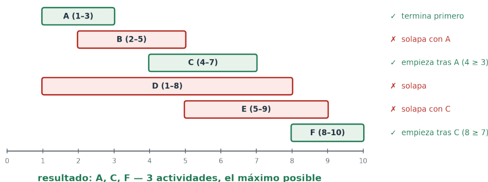
Figura 10.4: Selección de actividades: ordenadas por hora de fin, se acepta cada una que empiece después de la última aceptada. Resultado: A, C, F — el máximo posible (3).
