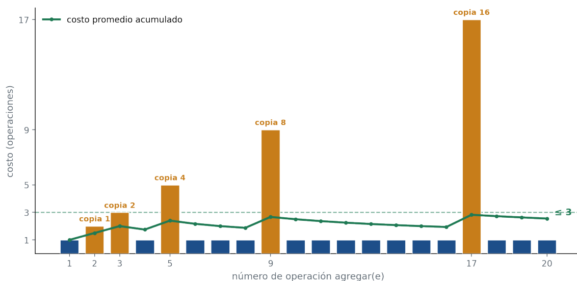
Figura 4.10: El costo de cada operación agregar con redimensión por duplicación. Casi todas cuestan 1 (azul); las que caen justo en una redimensión (naranja) pagan además la copia de todo lo existente. La línea verde —el promedio acumulado— nunca supera 3.
