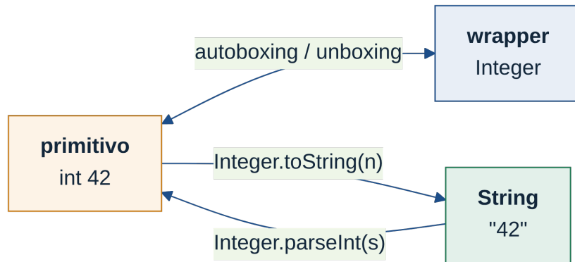
Figura 1B.8: El “triángulo” de conversiones: primitivo, wrapper y texto.
