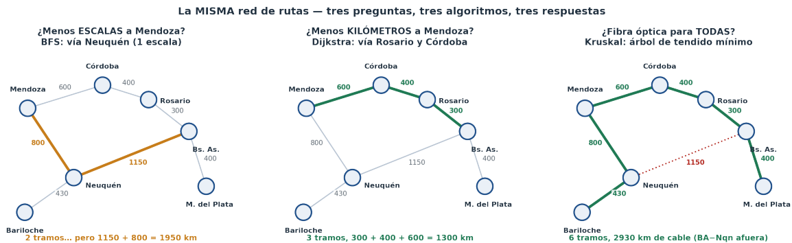
Figura 11.12: La misma red, tres preguntas. Izquierda: BFS minimiza tramos — a Mendoza por Neuquén, 1 escala, pero 1950 km. Centro: Dijkstra minimiza kilómetros — por Rosario y Córdoba, 3 tramos pero 1300 km. Derecha: Kruskal conecta las 7 ciudades con 2930 km de fibra, descartando la ruta más redundante (BA-Neuquén).
