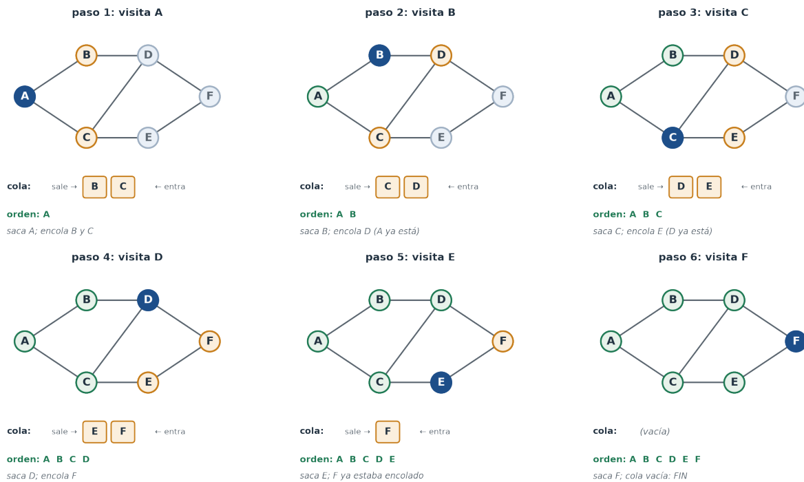
Figura 11.3: BFS paso a paso desde A. En cada paso: azul = el que se está visitando (recién salió de la cola), naranja = descubierto y esperando en la cola, verde = ya visitado. El orden final es A B C D E F.
