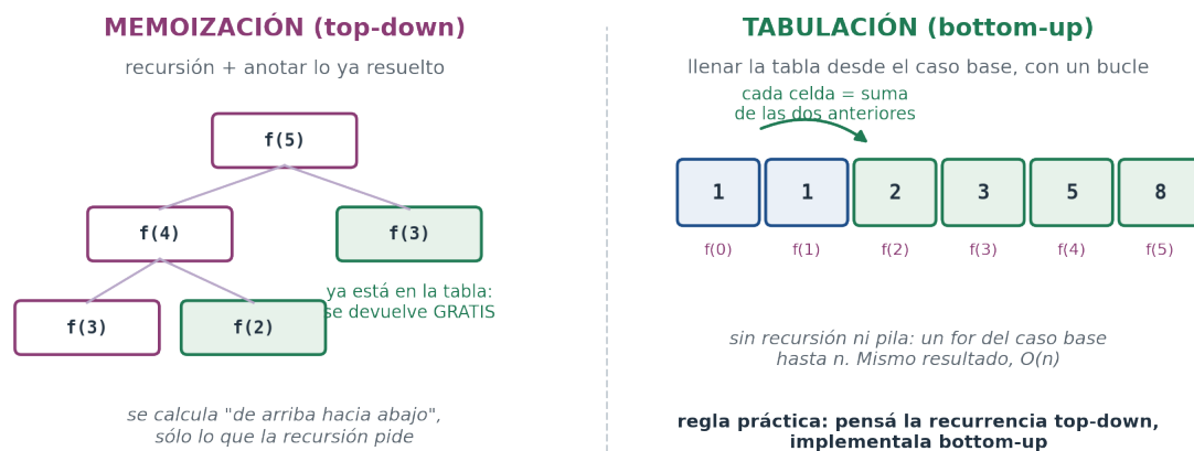
Figura 10.5: Memoización (top-down): la recursión natural más una tabla que evita recalcul — los subproblemas repetidos se devuelven gratis. Tabulación (bottom-up): un bucle llena la tabla desde el caso base. Regla práctica: pensá la recurrencia top-down, implementala bottom-up.
