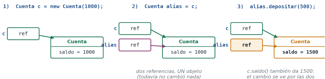
Figura 2.6: Aliasing en tres pasos: al asignar alias = c no se crea otra cuenta, sólo otra flecha. Depositar por alias cambia el único objeto, y c ve el nuevo saldo.
