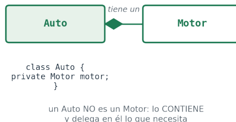
Figura 3.7: Herencia vs composición: Perro extends Animal porque un perro ES un animal; Auto tiene un campo Motor porque un auto TIENE un motor (en UML, el rombo lleno del lado del todo).
