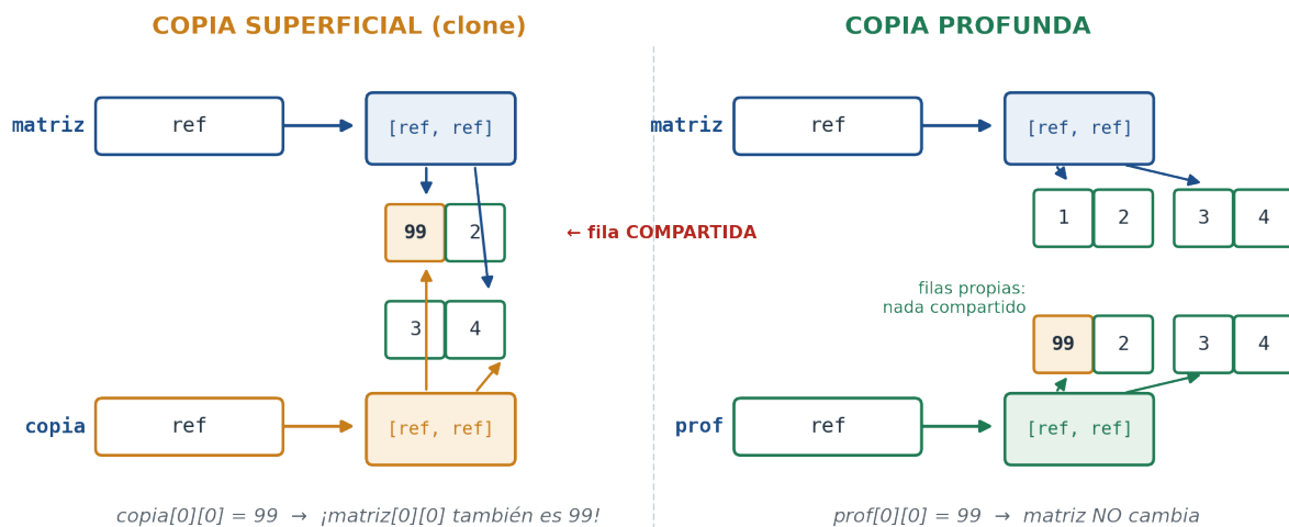
Figura 2.9: Copia superficial vs profunda de una matriz. Izquierda: clone() copia sólo el arreglo exterior; las filas quedan compartidas, y mutar copia[0][0] cambia también matriz[0][0] . Derecha: la copia profunda duplica también las filas; nada queda compartido.
