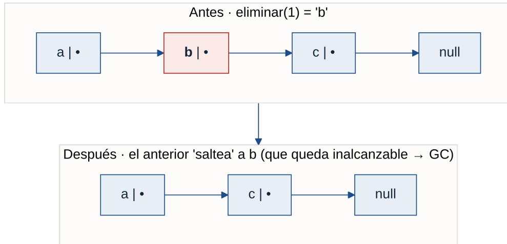
Figura 5.14: Eliminar: el nodo anterior saltea al que se elimina.
