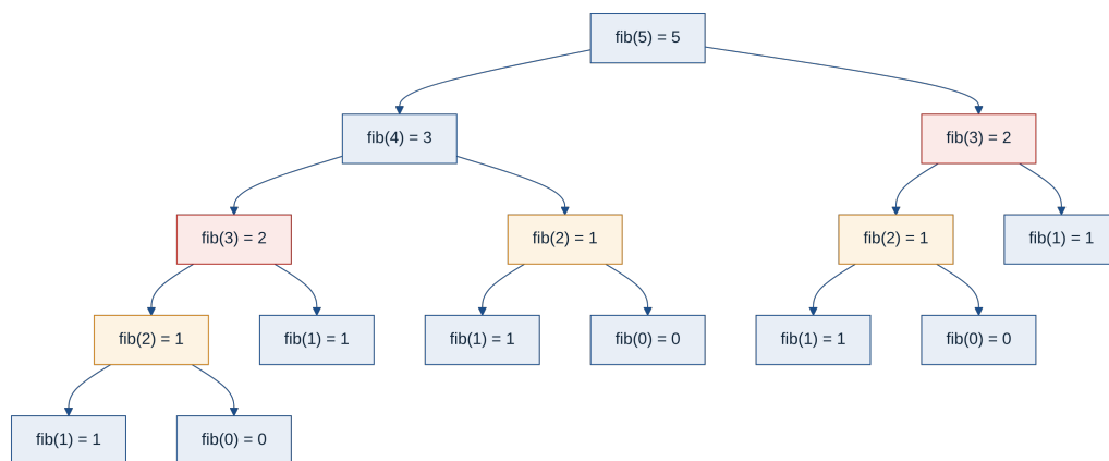
Figura 6.2: Árbol de llamadas de fib(5) con sus valores de retorno: fib(3) se calcula 2 veces (rojo) y fib(2) 3 veces (naranja). Cada subárbol repetido es trabajo hecho de nuevo.
