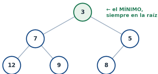
Figura 9.2: El invariante de min-heap: cada padre \leq sus hijos. No hay ningún orden entre hermanos: es una condición más débil que la del ABB, y por eso es más barata de mantener.
