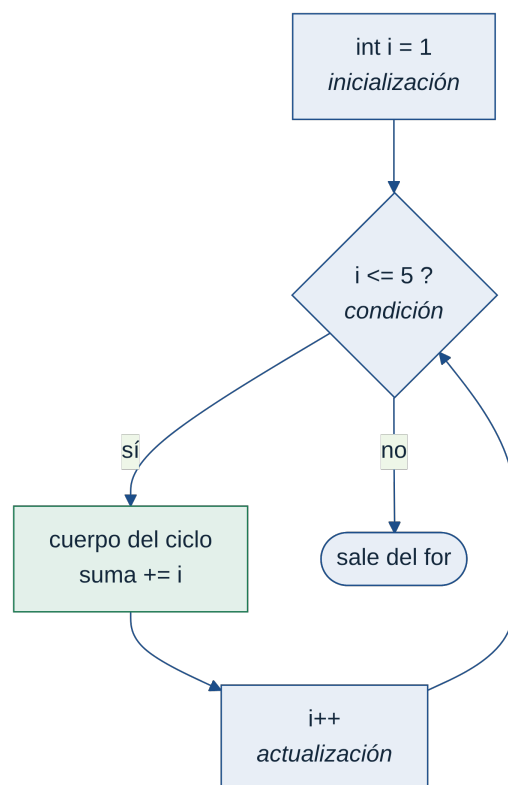
Figura 1B.11: Las tres partes del for y cómo se repite el ciclo.
