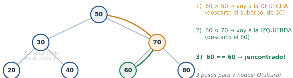
Figura 8.3: Buscar 60: tres comparaciones, cada una descarta medio árbol. El costo es O(\text{altura}) .
