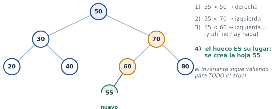
Figura 8.4: Insertar 55: desciende 50 → 70 → 60, y al no encontrar nada a la izquierda del 60, ahí mismo se engancha. El invariante se preserva solo.
