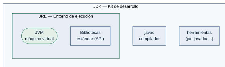
Figura 1B.4: El JDK contiene todo lo necesario para desarrollar; adentro, el JRE contiene lo necesario para ejecutar.
