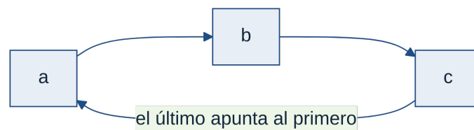
Figura 5.18: En la lista circular, el último nodo apunta de nuevo al primero.
