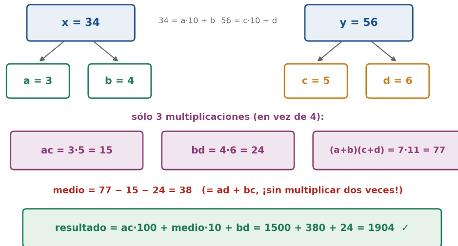
Figura 6.7: Karatsuba con 34 \times 56 : se parte cada número en dos mitades, se hacen sólo tres multiplicaciones chicas, y el término del medio se obtiene restando.
