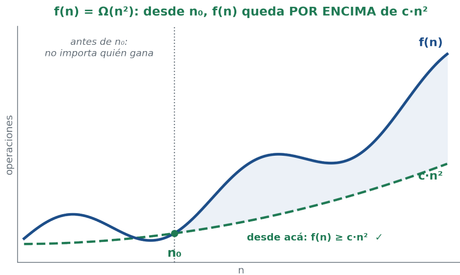
Figura 4.4: Cota inferior: desde su propio n_0 (fíjate que no es el mismo que el de la figura anterior), f(n) nunca vuelve a caer por debajo de c \cdot n^2 .
