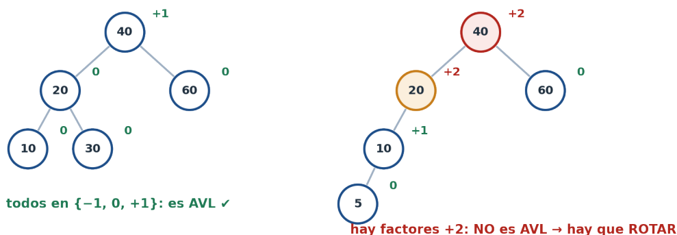
Figura 8.8: El factor de equilibrio en cada nodo. El AVL exige -1, 0 o +1 en todos; un +2 o -2 dispara una rotación.
