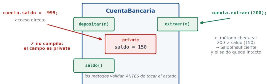
Figura 3.4: Encapsulamiento: el campo saldo es privado, así que el acceso directo ni siquiera compila. La única forma de tocar el estado son los métodos, que validan antes de modificar.
