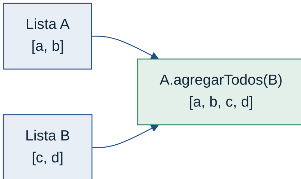
Figura 5.6: agregarTodos : los elementos de la otra lista se agregan al final, en orden.
