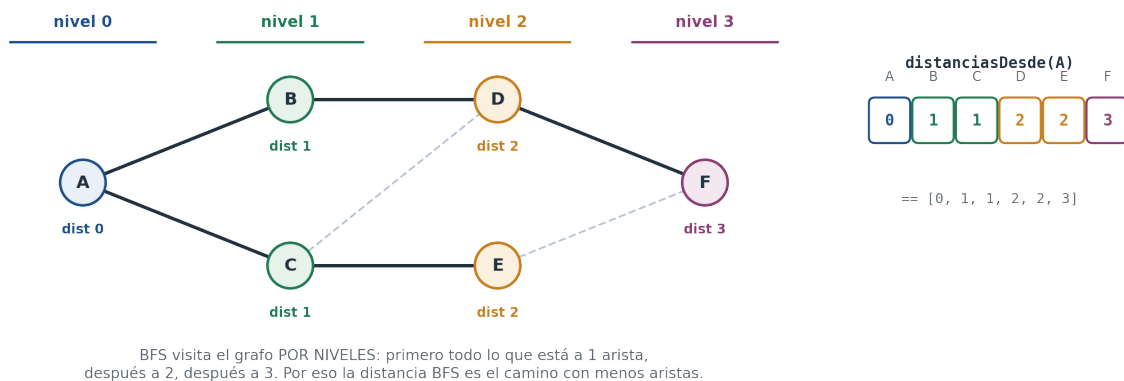
Figura 11.4: El mismo grafo estirado por niveles. Las aristas oscuras son las que BFS usó para descubrir cada vértice; las punteadas existen pero no descubrieron a nadie. La distancia de cada vértice es su nivel — el arreglo que devuelve distanciasDesde(A) .
