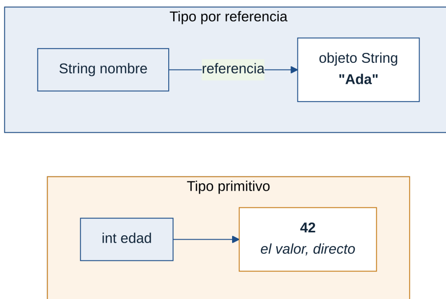
Figura 1B.7: Un primitivo guarda el valor; una referencia “apunta” a un objeto en memoria.
