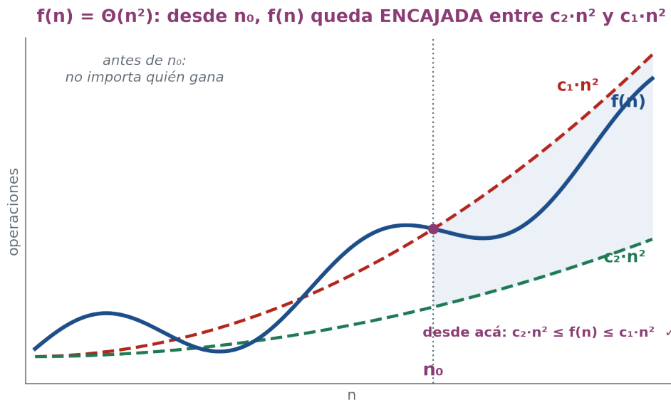
Figura 4.5: Cota ajustada: desde n_0 , f(n) queda “encajada” para siempre entre c_2 \cdot n^2 y c_1 \cdot n^2 .
