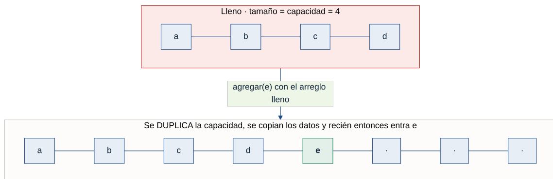
Figura 5.2: Cuando el arreglo se llena, se duplica la capacidad y se copian los datos.
