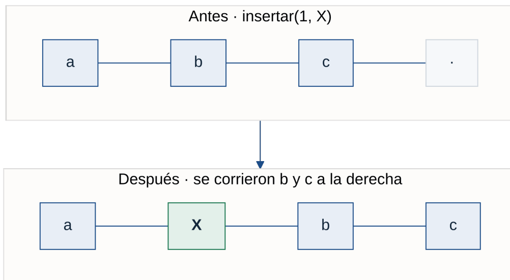
Figura 5.3: insertar(1, X): hay que correr b y c una posición a la derecha.
