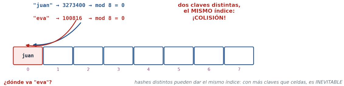
Figura 7.4: Una colisión real: "juan" y "eva" tienen hashCodes distintos (3273400 y 100816), pero ambos dan índice 0 en una tabla de 8 celdas. ¿Dónde va la segunda?
