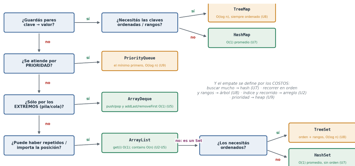
Figura 12.2: Cuatro preguntas bastan: ¿clave→valor? ¿prioridad? ¿sólo extremos? ¿repetidos? — y el desempate final entre hash ( O(1) , sin orden) y árbol ( O(\log n) , con orden).
