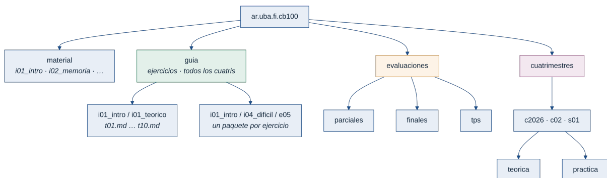
Figura 1B.20: Esquema de paquetes del repositorio único de la materia.
