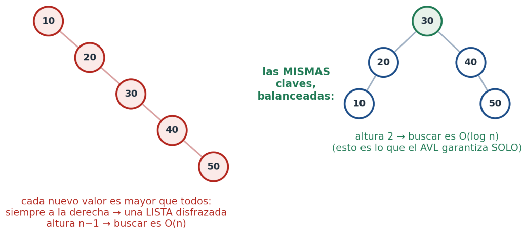
Figura 8.7: Insertar 10, 20, 30, 40, 50 en orden produce una “lista disfrazada” de altura n-1 : buscar vuelve a ser O(n) . Las mismas claves, balanceadas, tienen altura 2.
