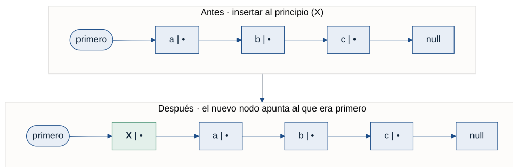
Figura 5.13: Insertar al principio: el nuevo nodo apunta al viejo primero, sin mover el resto.
