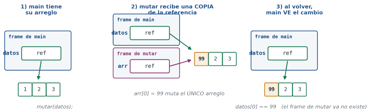
Figura 2.7: Mutar a través del parámetro: arr es una copia de la referencia de datos, pero ambas llevan al mismo arreglo. La mutación sobrevive al método.
