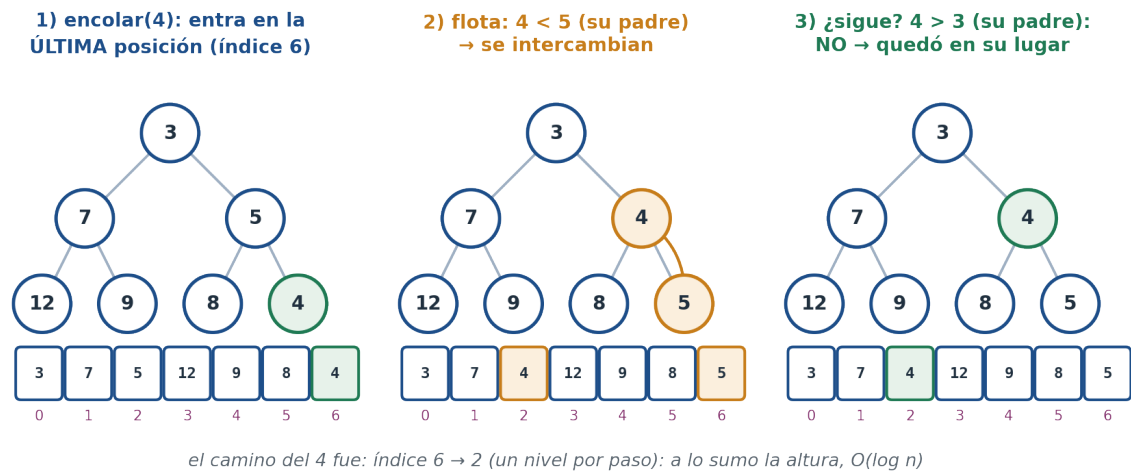
Figura 9.3: Encolar 4, paso a paso: entra en la última posición (índice 6), flota intercambiándose con su padre 5, y se detiene al encontrar un padre menor (3). Cada intercambio sube un nivel: O(\log n) .
