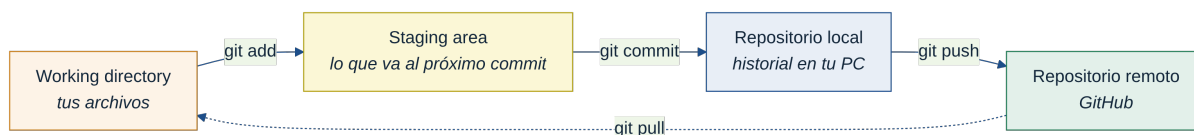
Figura 1B.6: El flujo básico de Git: tus cambios pasan del working directory al staging y de ahí a un commit en el repositorio.
