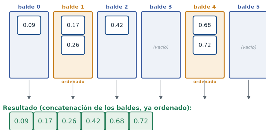
Figura 6.10: Bucket sort, Pasos 2 y 3: se ordena cada balde por dentro (resaltados los que se reordenan) y luego se concatenan los baldes en orden para obtener el arreglo final ordenado.
