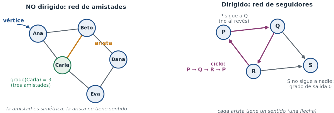
Figura 11.1: A la izquierda, un grafo NO dirigido: la amistad va en ambos sentidos y las aristas son simples líneas. A la derecha, uno dirigido: “P sigue a Q” no implica que Q siga a P, y las aristas son flechas. El ciclo P \rightarrow Q \rightarrow R \rightarrow P está resaltado.
