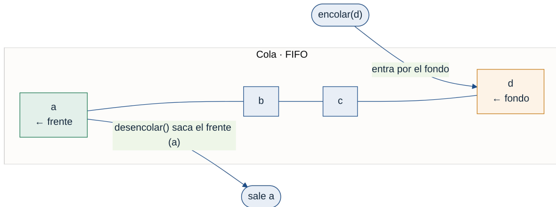
Figura 5.24: La cola entra por el fondo y sale por el frente: FIFO.
