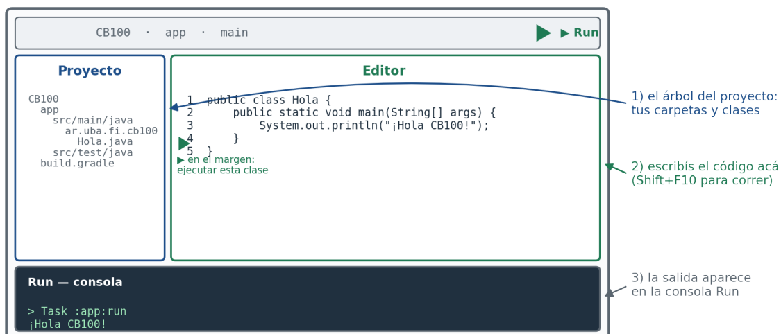
Figura 1B.5: Esquema de la ventana de IntelliJ: árbol del proyecto, editor con el botón de ejecución en el margen, y consola Run con la salida.
