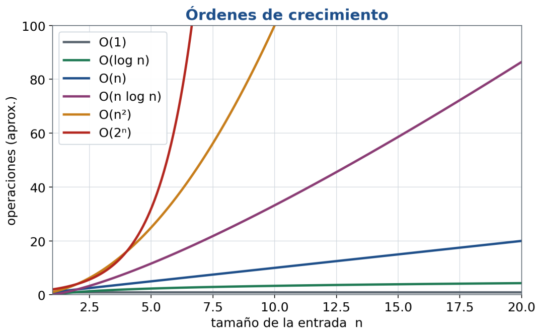
Figura 4.2: Cómo crecen los distintos órdenes. Un algoritmo O(2^n) o O(n^2) se vuelve impracticable enseguida.
