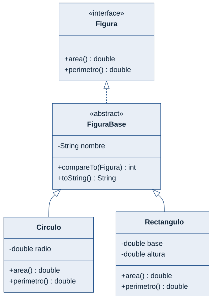
Figura 3.9: El TDA Figura (interfaz), la clase abstracta FiguraBase y las figuras concretas.
