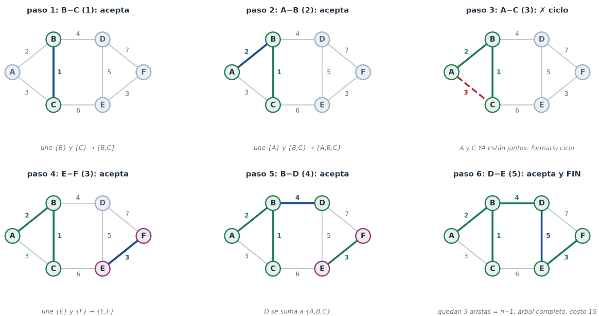
Figura 11.9: Kruskal sobre la red de ejemplo. Las aristas se procesan ordenadas por peso: 1, 2, 3, 3, 4, 5. El color de cada vértice indica su grupo. La única rechazada es A–C (3): A y C ya estaban en el mismo grupo verde y cerrarían un ciclo. Con 5 aristas aceptadas ( n-1 ) el árbol está listo: costo 15.
