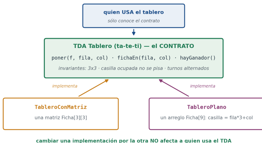
Figura 3.1: El TDA como contrato: quien usa el Tablero conoce sólo sus operaciones y sus invariantes. Abajo, dos implementaciones intercambiables — matriz o arreglo plano —: cambiar una por otra no afecta al usuario.
