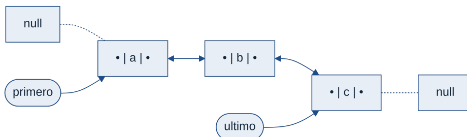
Figura 5.15: Cada nodo conoce a su anterior y a su siguiente.
