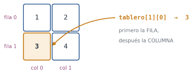
Figura 1B.14: Una matriz es un arreglo de arreglos: tablero[1][0] es el elemento de la fila 1, columna 0.
