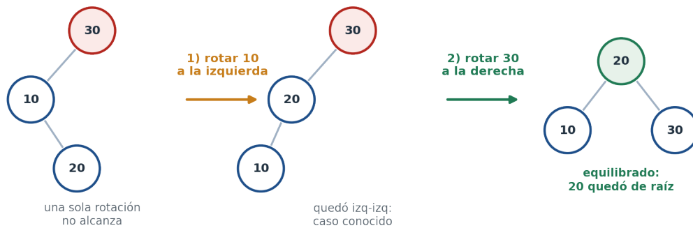
Figura 8.10: La rotación doble (caso izq-der) con el ejemplo mínimo 30, 10, 20: primero se rota 10 a la izquierda (queda izq-izq), después 30 a la derecha. El del medio (20) termina de raíz.
