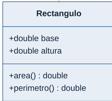
Figura 1B.15: Diagrama UML de la clase Rectangulo: sus campos y sus métodos.
