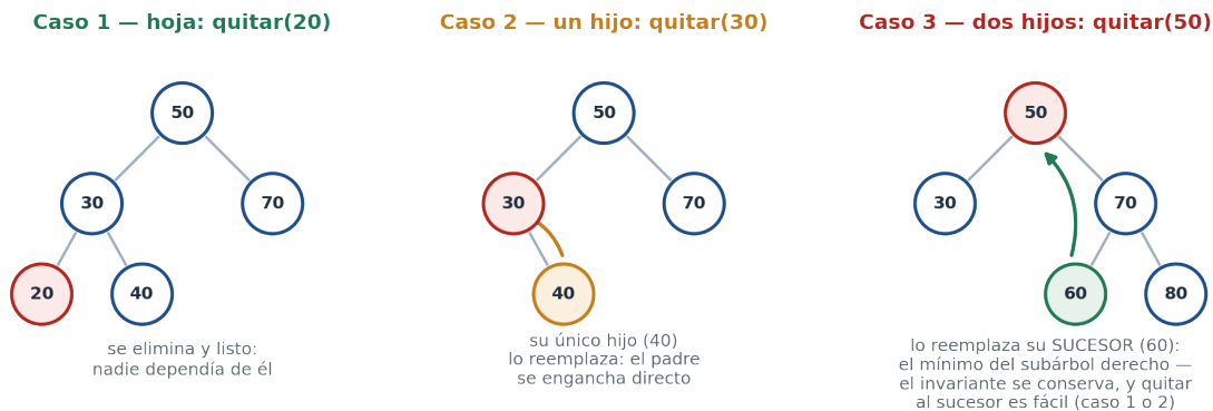
Figura 8.5: Los tres casos de quitar: la hoja se elimina y listo; el nodo con un hijo es reemplazado por ese hijo; el nodo con dos hijos es reemplazado por su sucesor (el mínimo del subárbol derecho).
