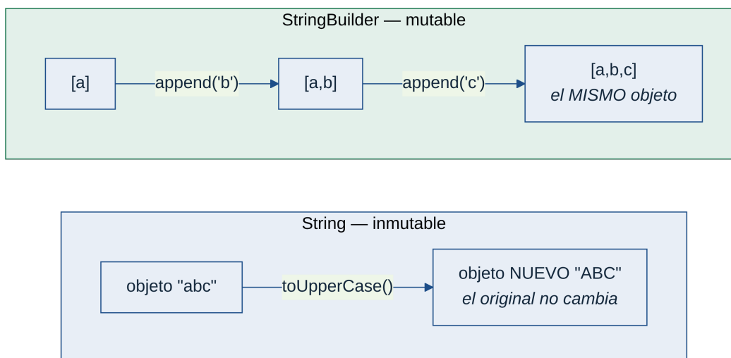
Figura 1B.9: El String es inmutable (cada método crea uno nuevo); el StringBuilder es mutable (modifica el mismo objeto).
