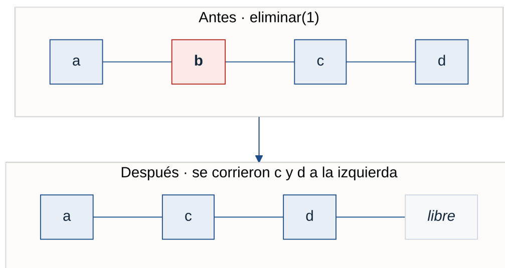
Figura 5.4: eliminar(1): se corren c y d a la izquierda para tapar el hueco.
