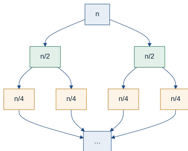
Figura 4.6: Árbol de recursión de T(n) = 2T(n/2) + n : cada nivel suma n ; hay \log_2 n niveles.
