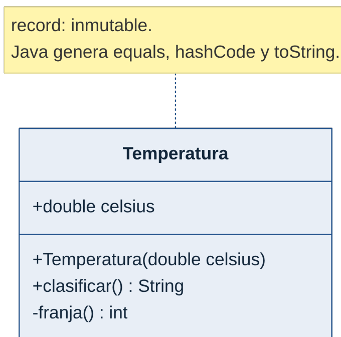
Figura 1B.16: Diagrama UML de la clase Temperatura. El + indica visibilidad pública; el -, privada.
