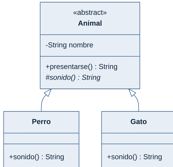
Figura 3.5: Herencia: Perro y Gato son Animal; heredan presentarse() y definen su sonido().
