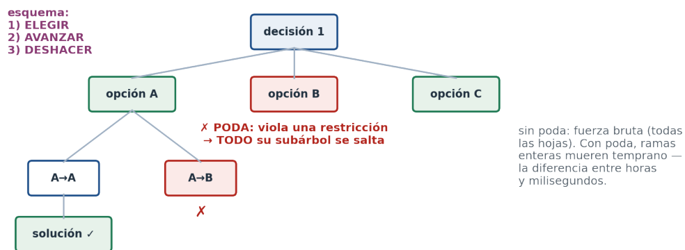
Figura 10.1: El backtracking recorre el árbol de decisiones en profundidad. La poda descarta subárboles enteros apenas se viola una restricción — la diferencia entre horas y milisegundos.
