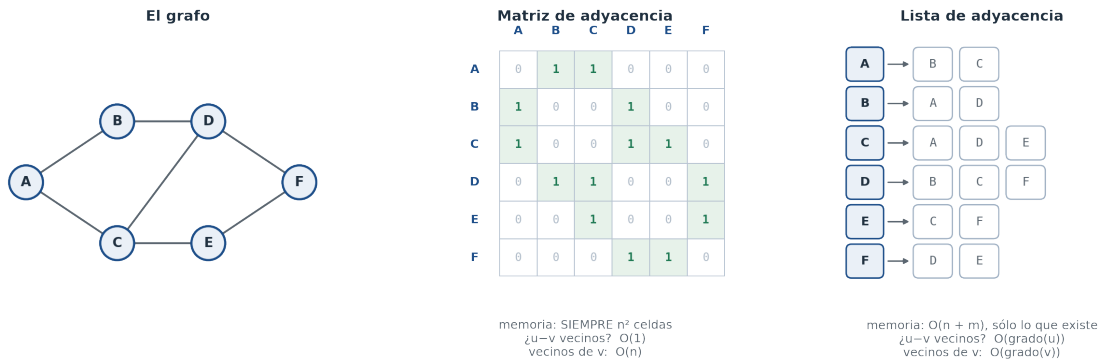
Figura 11.2: El mismo grafo tres veces: el dibujo, la matriz de adyacencia (una tabla n \times n con 1 donde hay arista) y la lista de adyacencia (cada vértice con la lista de sus vecinos). La matriz gasta n^2 celdas aunque casi todas tengan 0; la lista guarda sólo lo que existe.
