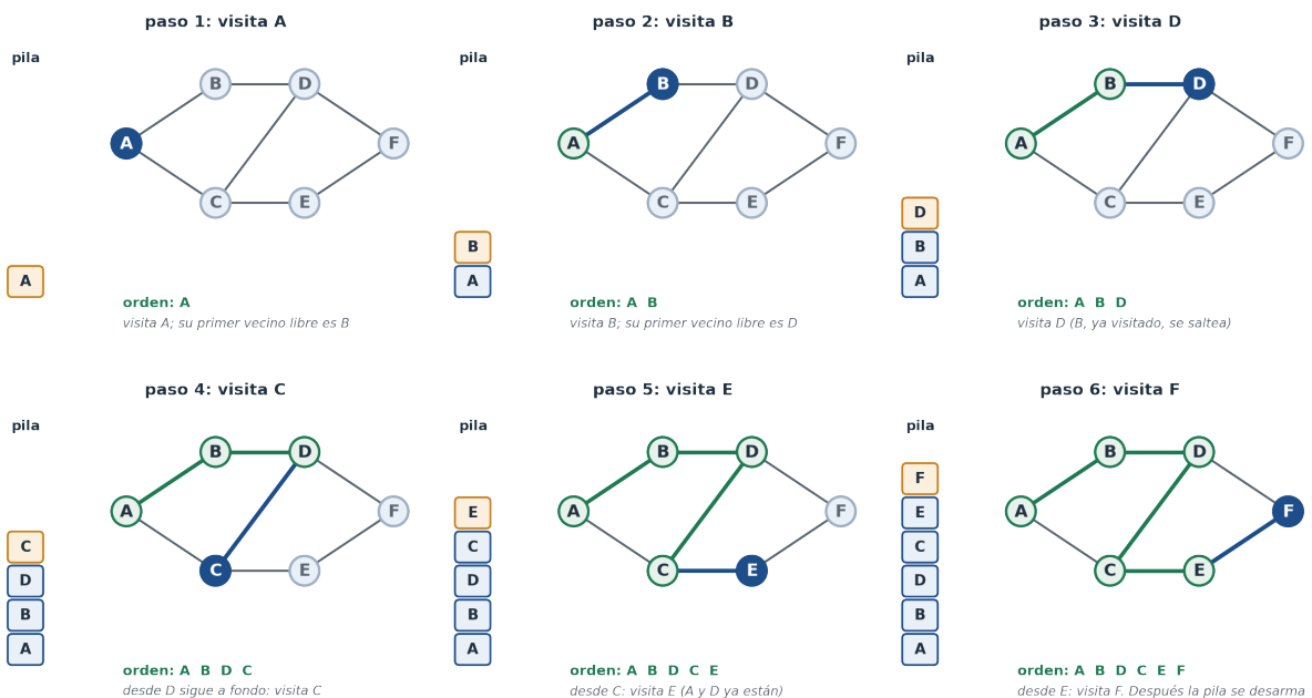
Figura 11.5: DFS paso a paso desde A. La pila de llamadas crece a la izquierda de cada panel: A llama a B, B llama a D, D llama a C... El recorrido “serpentea” hasta el fondo: A B D C E F. Azul = arista por la que acaba de meterse; verde = camino ya recorrido.
