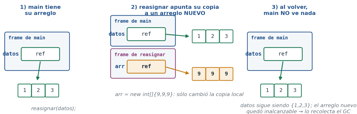
Figura 2.8: Reasignar el parámetro: la copia local apunta a otro arreglo, pero la referencia original de main no cambia. El arreglo nuevo muere con el método.
