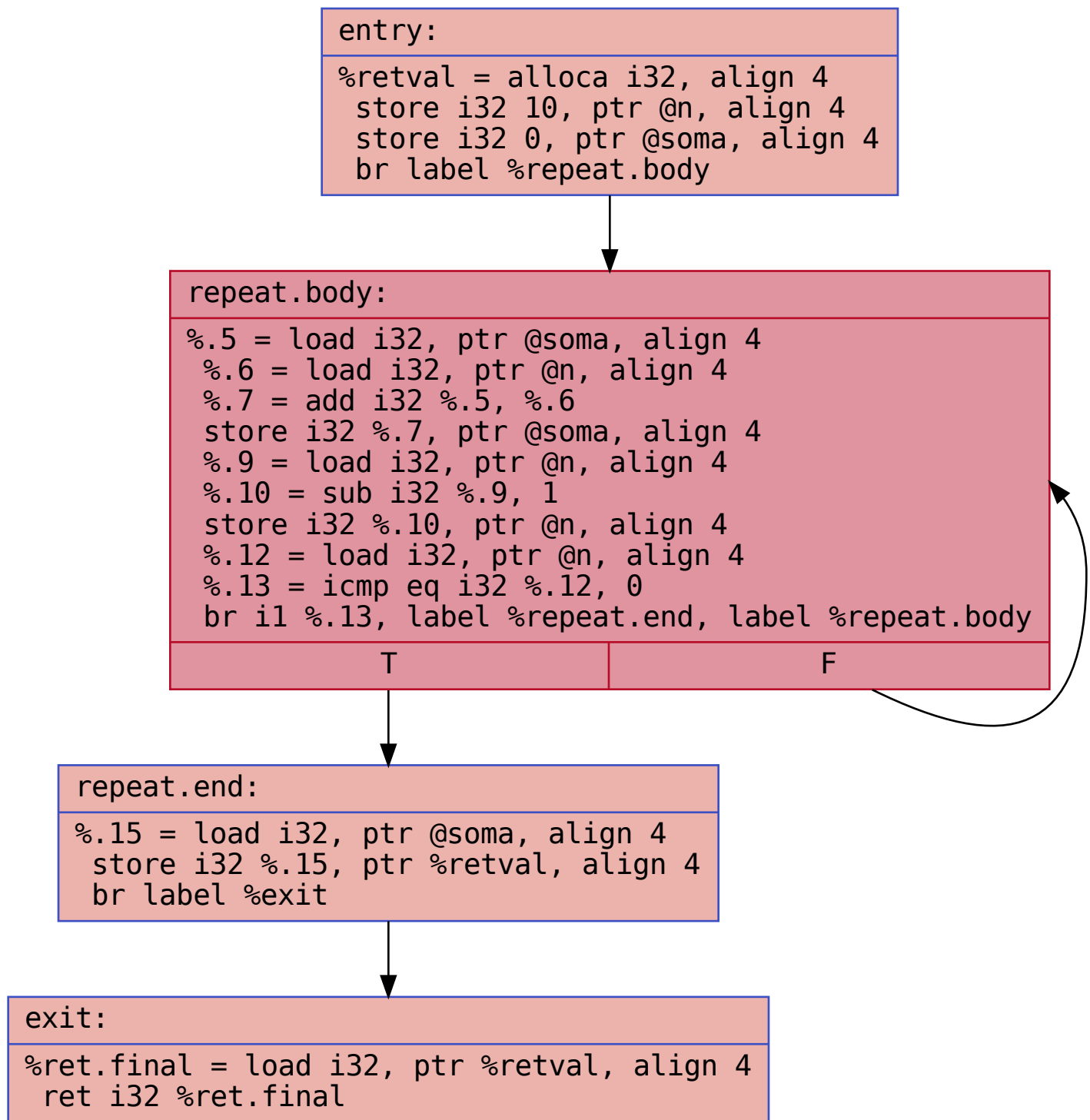
CFG for 'main' function
