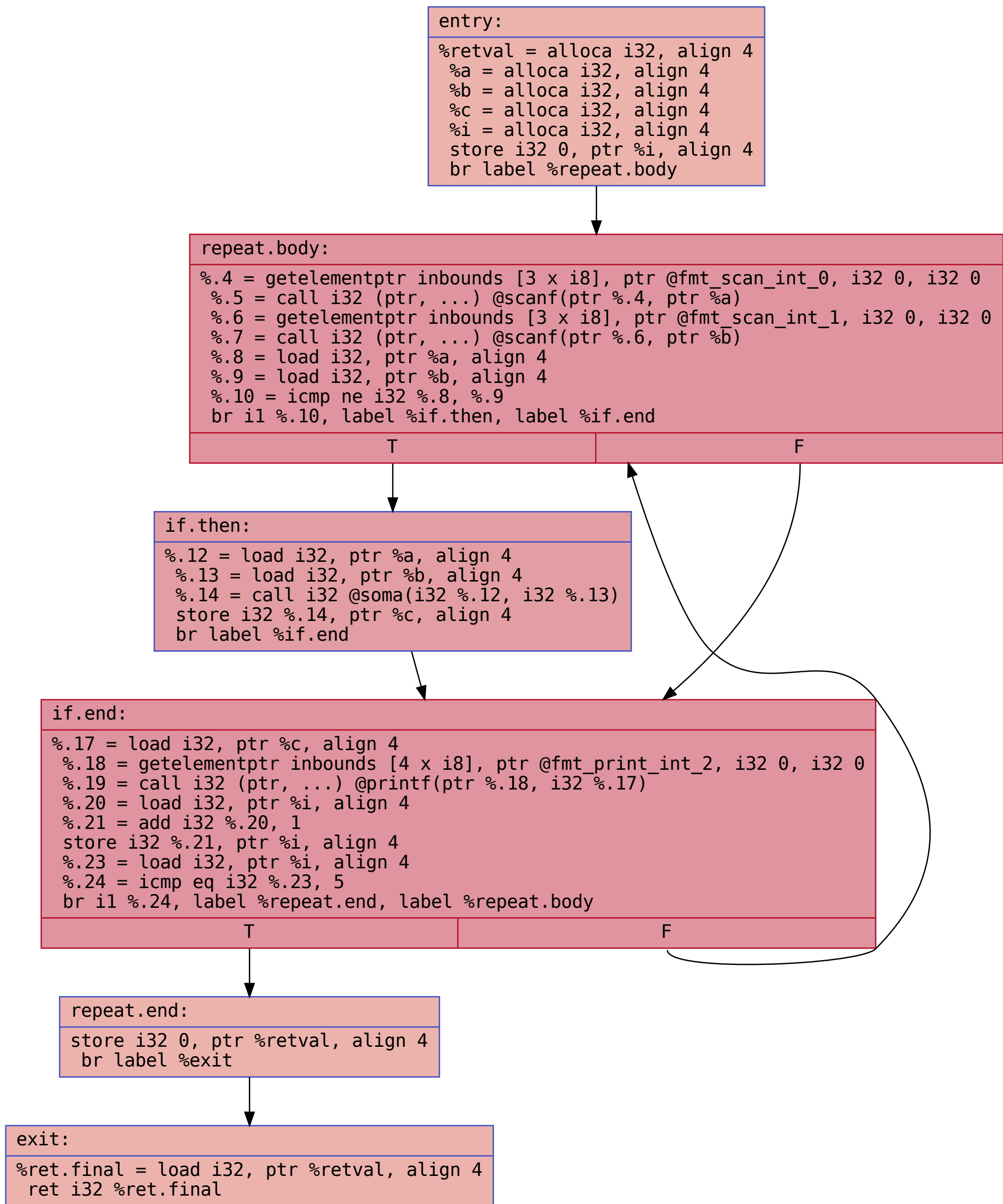
CFG for 'main' function
