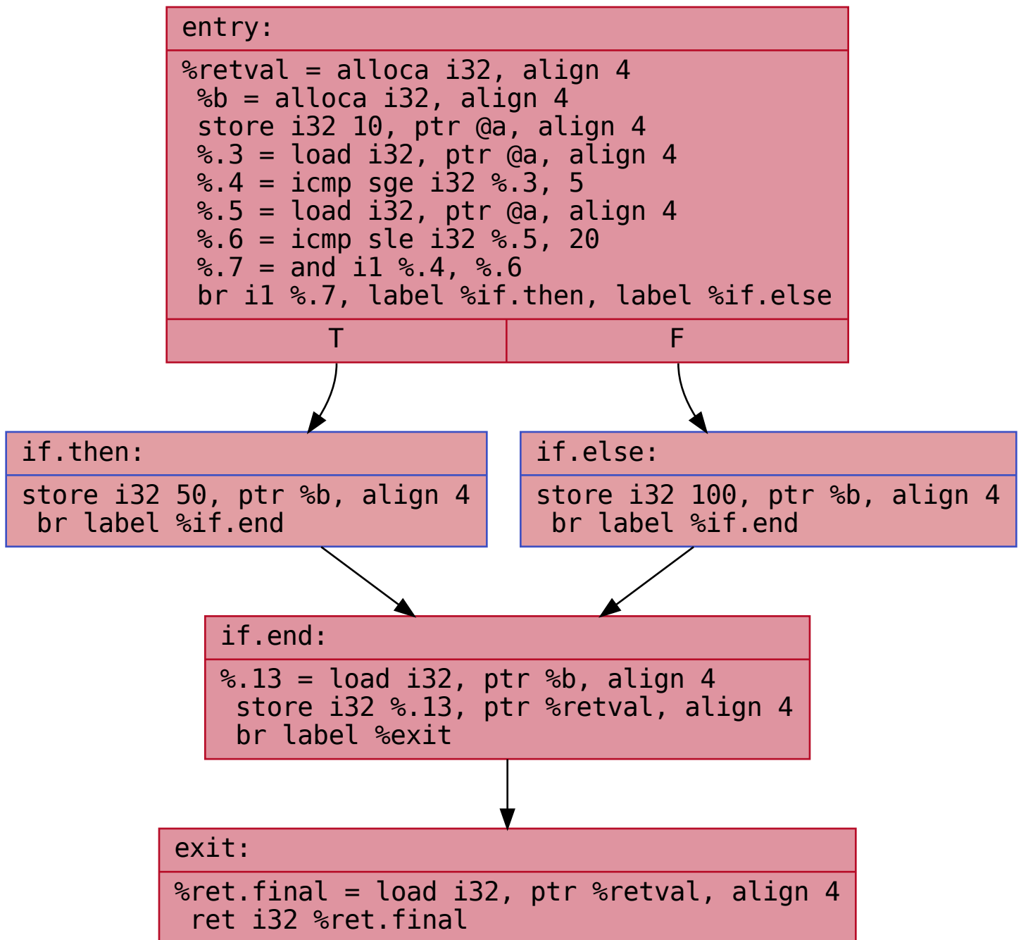
CFG for 'main' function
