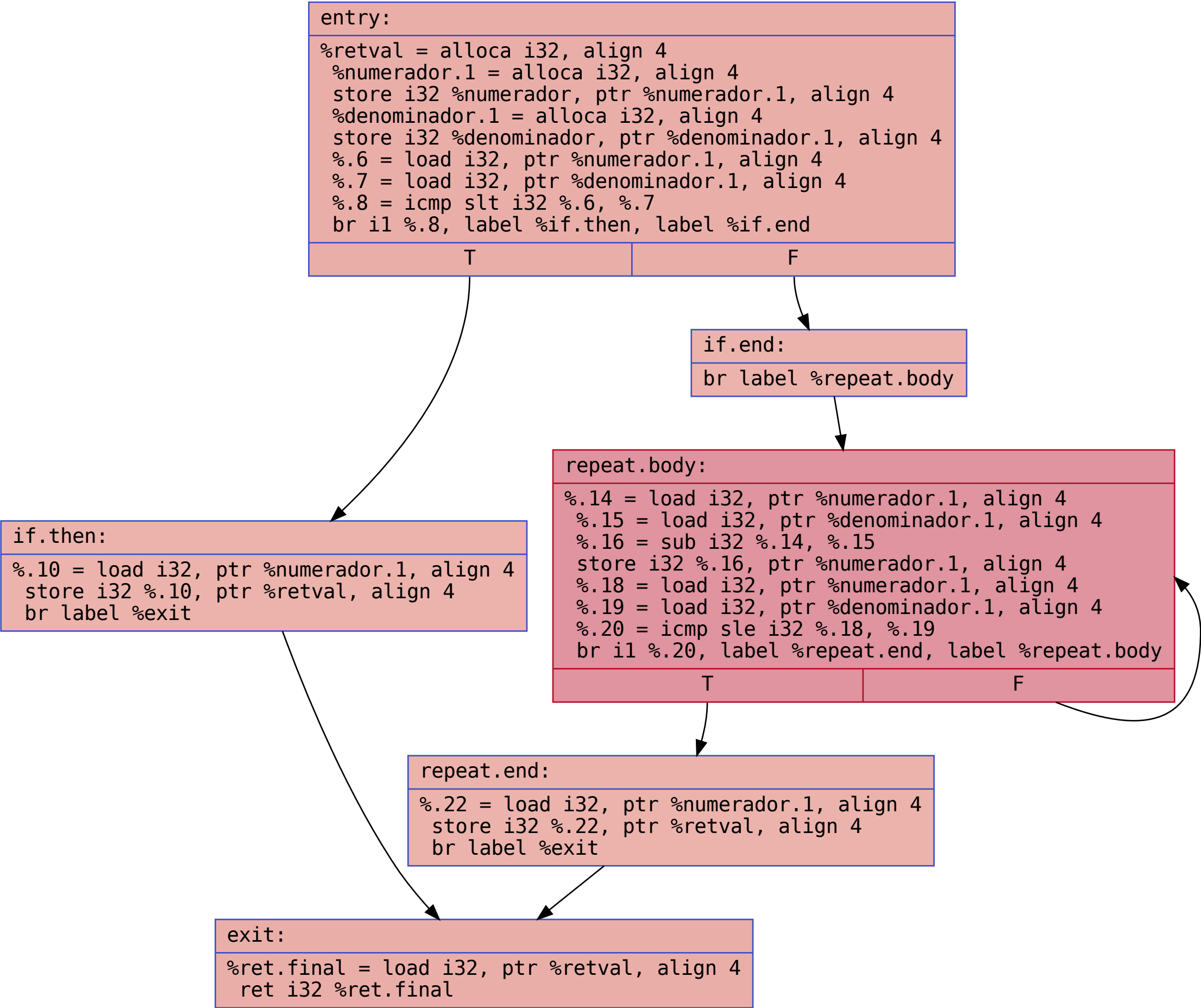
CFG for 'modulo' function
