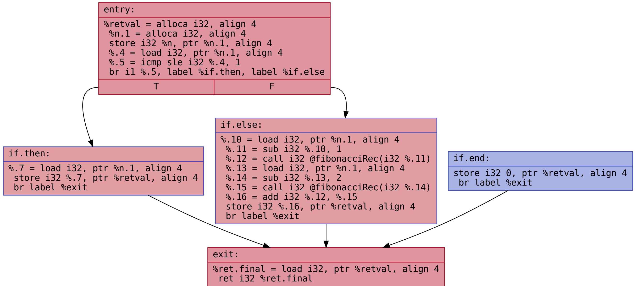
CFG for 'fibonacciRec' function
