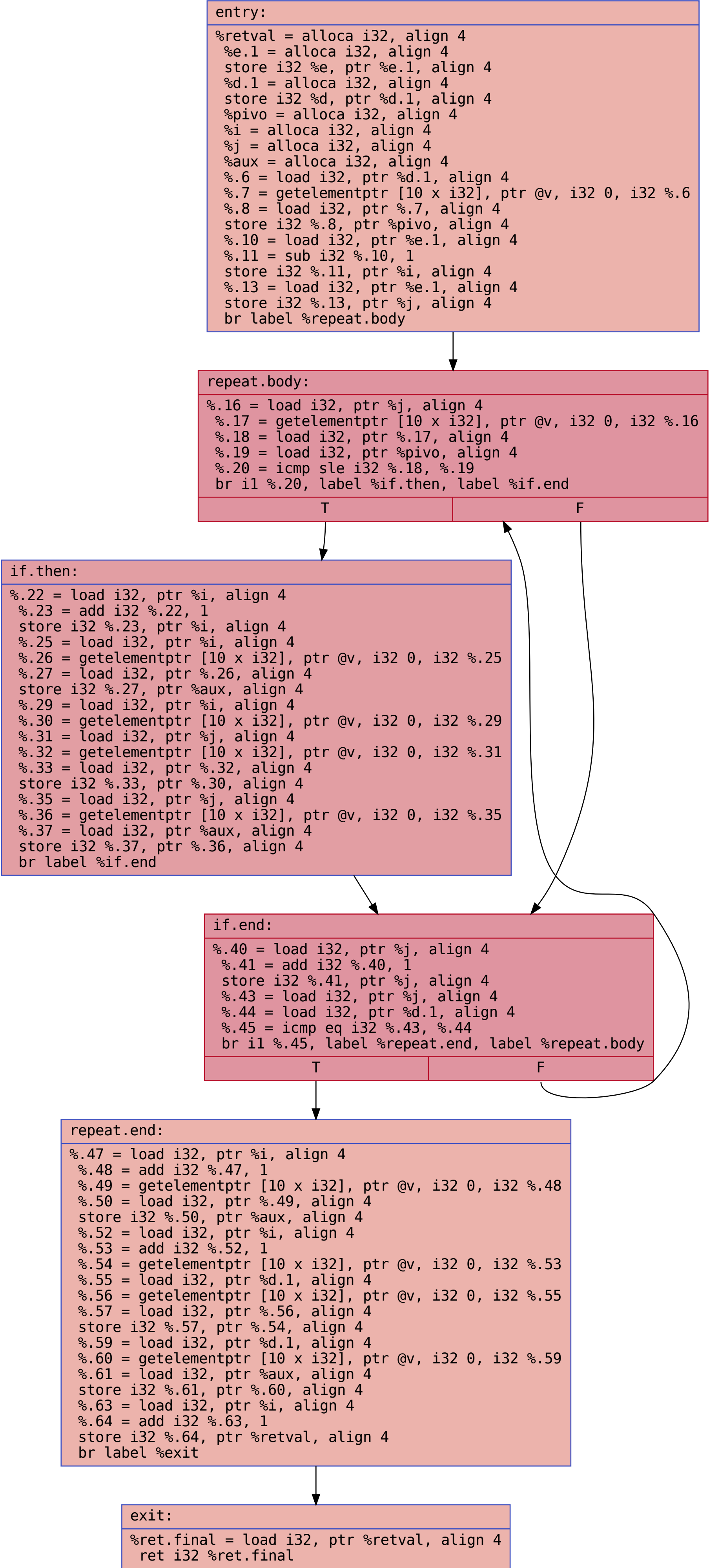
CFG for 'partition' function
