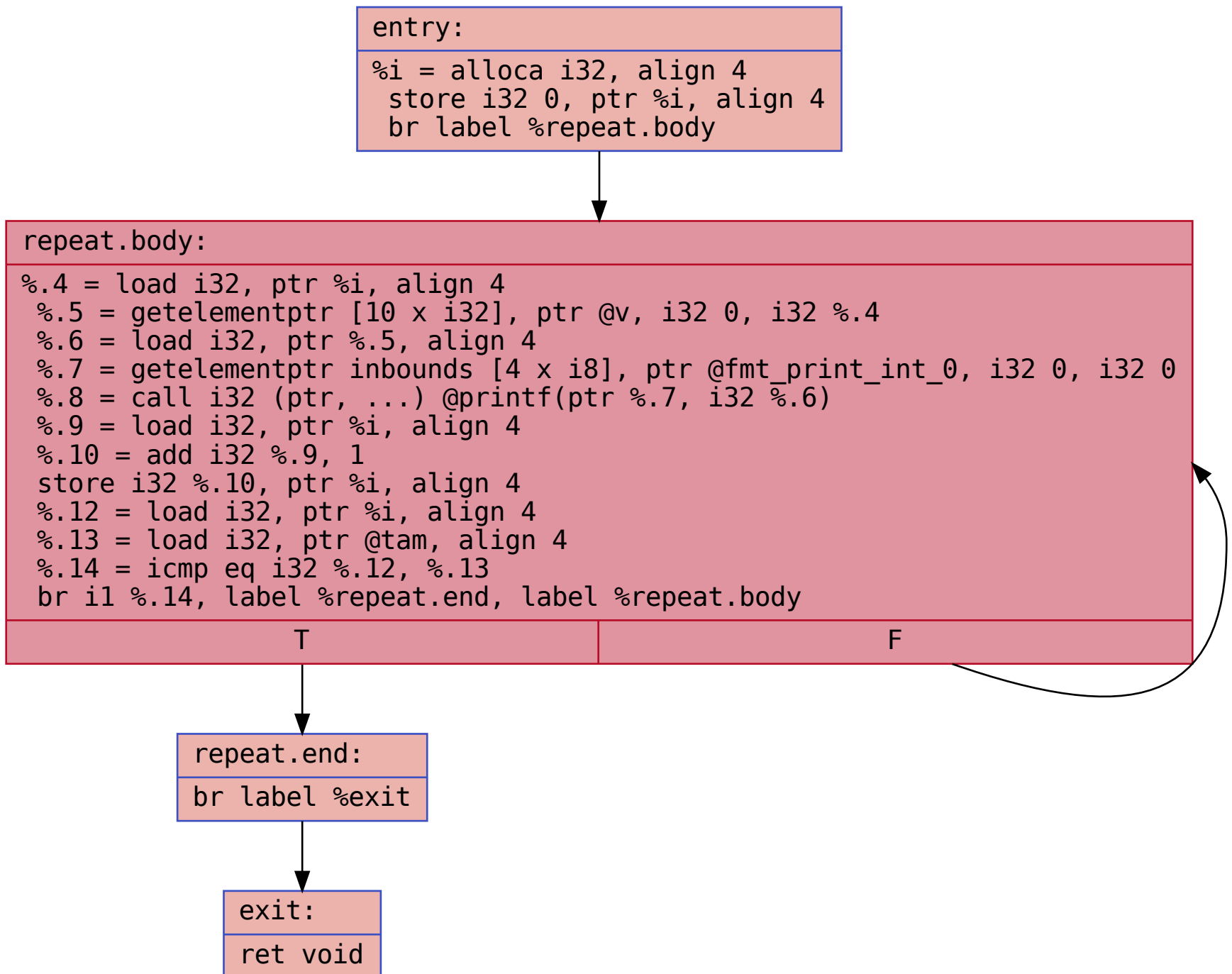
CFG for 'printArray' function
