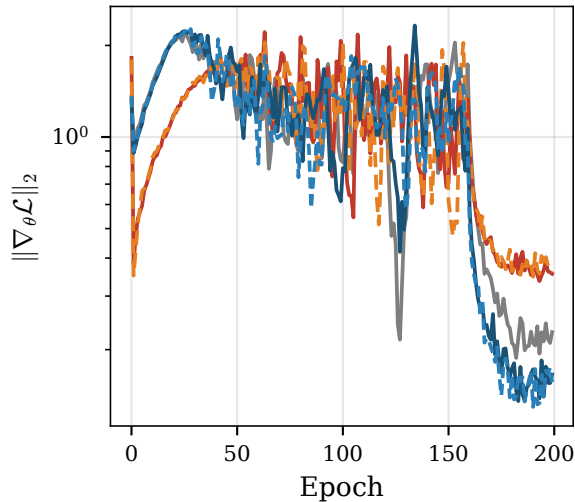
(b) Gradient norm
