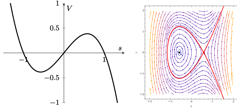
FIGURA 9. Potenziale nell'Esempio ?? e piano delle fasi associato con rappresentazione del flusso di fase. Sono indicati i punti critici e le separatrici (in rosso) per un punto materiale di massa m = 1 .
