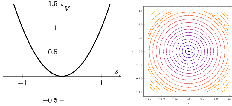
FIGURA 7. Potenziale e piano delle fasi associato con rappresentazione del flusso di fase relativo all'esempio ??.
