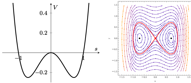
FIGURA 8. Potenziale nell'Esempio ?? e piano delle fasi associato con rappresentazione del flusso di fase. Sono indicati i punti critici e le separatrici (in rosso) per un punto materiale di massa m = 1 .
