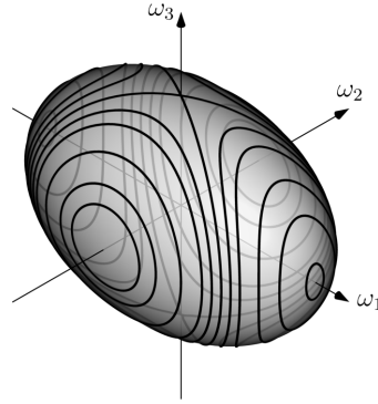
FIGURA 3. Poloidi sull'ellissoide di inerzia \langle \boldsymbol{\omega}, \mathbf{I}_O(\boldsymbol{\omega}) \rangle = 2E .
