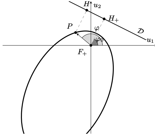
FIGURA 3. Conica in forma polare.
