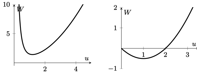
FIGURA 1. Potenziale W nel teorema di Bertrand per b = 2 (sinistra) e b = -1 (destra) con \bar{a} = 1 .
