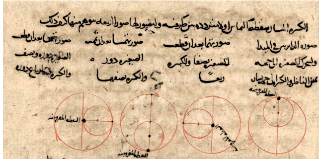
FIGURA 2. Schema di Tūsī per la cinematica nell'Esercizio E7.14, dal suo Commentario sulle scienze astronomiche ( al-Tadhkirah fi 'ilm al-hay'a ).
