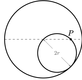
FIGURA 2. Schema di Tūsī per la cinematica nell'Esercizio E7.14, dal suo Commentario sulle scienze astronomiche ( al-Tadhkirah fi 'ilm al-hay'a ).
