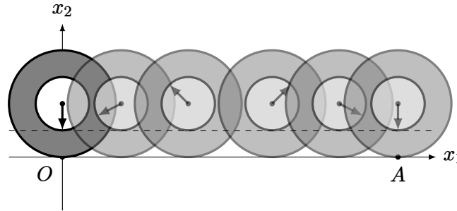
FIGURA 2. Schema di Tūsī per la cinematica nell'Esercizio E7.14, dal suo Commentario sulle scienze astronomiche ( al-Tadhkirah fi 'ilm al-hay'a ).
