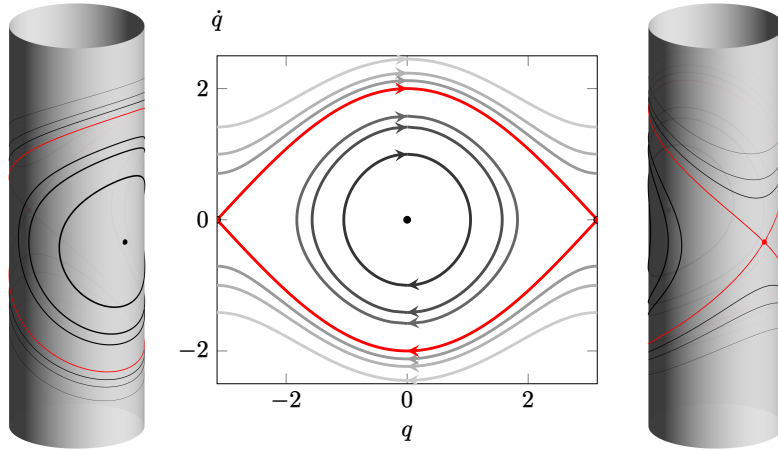
FIGURA 10. Piano delle fasi del pendolo con g/l = 1 . Sono visualizzate le traiettorie per diversi valori di e , inclusa la separatrice ( e = 1 , linea rossa) e i due punti critici stabile (nero) e instabile (rosso).
