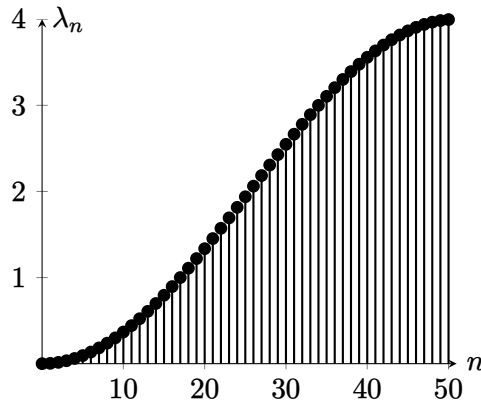
FIGURA 1. Autovalori della matrice tridiagonale simmetrica di Toeplitz con a = 2 e b = -1 .
