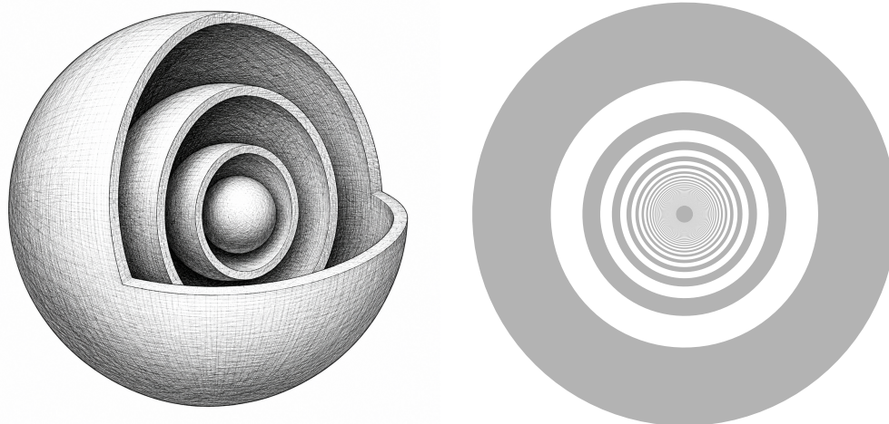
FIGURA 2. Uno schema della teoria, proposta da Edmund Halley nel 1692, di una Terra “a gusci”. La teoria aveva l’obiettivo di spiegare alcune anomalie del campo magnetico terrestre. A destra, la speciale progressione dell’Esercizio E5.6.
