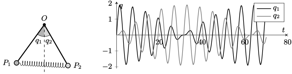
FIGURA 11. Problema dei pendoli accoppiati (sinistra). Fenomeno dei battimenti per 0 < k \ll 1 (destra).
