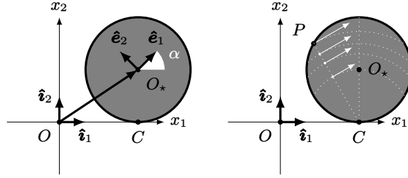
FIGURA 1. Anello che rotola di rotolamento puro. Il punto di contatto C è istantaneamente fermo ed è centro istantaneo di rotazione.
