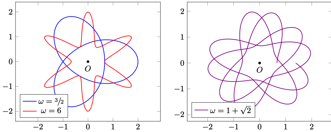
FIGURA 1. Orbite nell'Esercizio E5.5 per diversi valori di \omega . In tutti i casi, e = 1/2 . Orbite con \omega \in \mathbb{Q} sono chiuse, diversamente si ha a che fare con orbite aperte.
