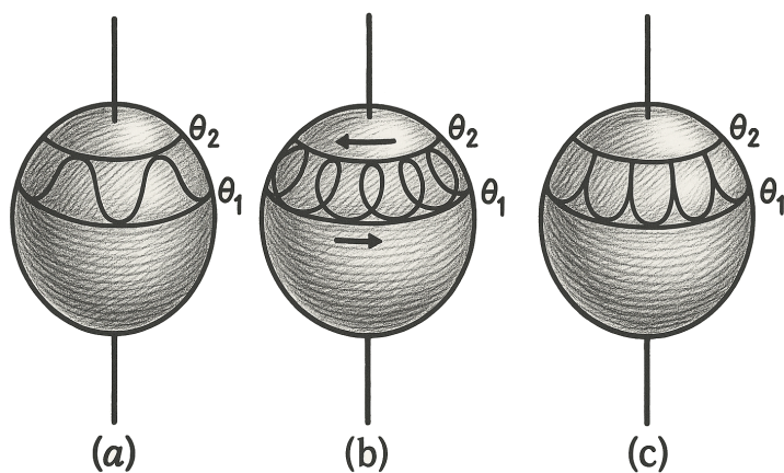
FIGURA 5. Moto di una trottola di Lagrange per diversi valori dei suoi parametri. Figura adattata dalla monografia Fisica teorica I. Meccanica di L.D. Landau e E.M. Lifšits (1976).
