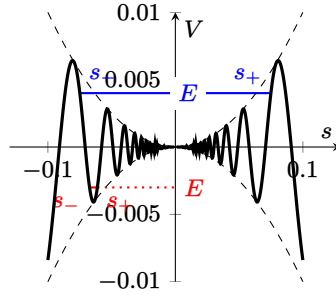
FIGURA 6. Potenziale nell'Esempio 2.11 e due intervalli ammessi per il moto per diversi valori di E .
