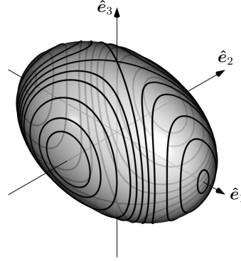
FIGURA 3. Poloidi sull'ellissoide \langle \boldsymbol{\omega}, \mathbf{I}_O \boldsymbol{\omega} \rangle = 2E .
