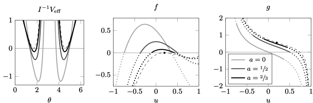
FIGURA 4. Esempio di grafico delle funzioni f e g e del potenziale efficace nella dinamica della trottola di Lagrange per 2\alpha = \beta = b = 1 . La linea tratteggiata corrisponde al caso limite in cui u_- \rightarrow u_+ .
