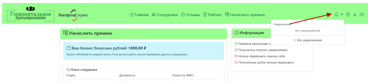
Рисунок 19 – Кнопка «Уведомления»
