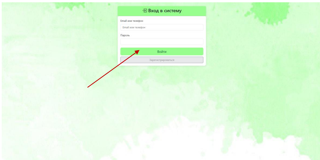
Рисунок 3 – Кнопка «Войти»
