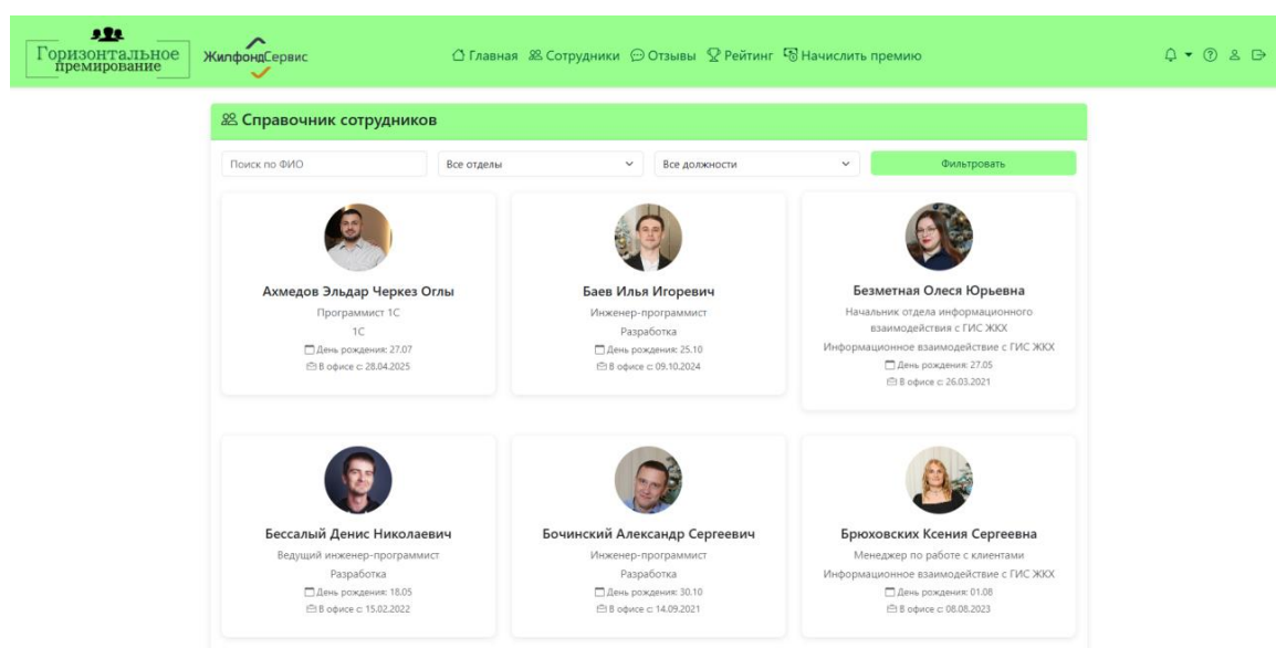
Рисунок 9 – Вкладка «Сотрудники»
