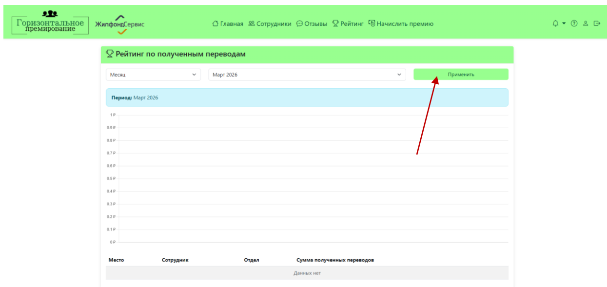
Рисунок 16 – Фильтрация рейтинга
