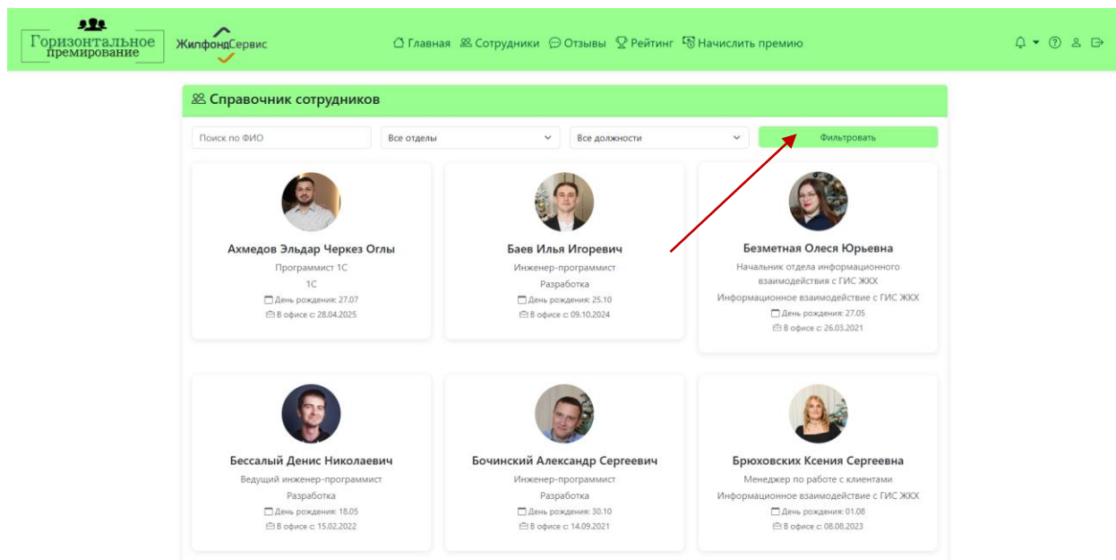
Рисунок 10 – Кнопка «Фильтровать»
