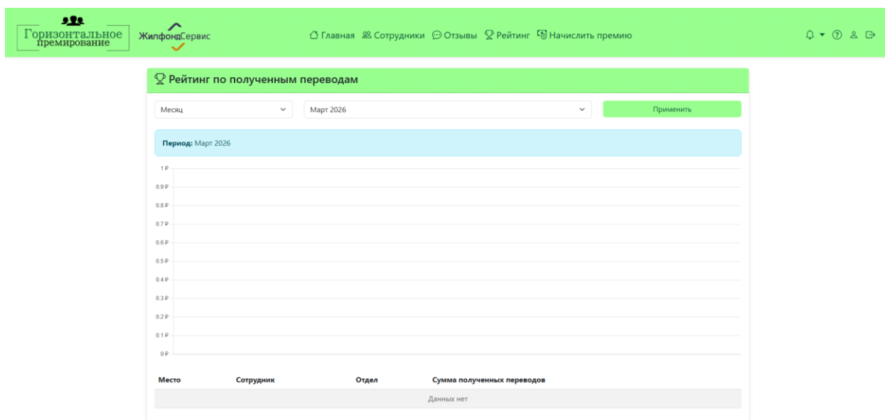
Рисунок 15 – Вкладка «Рейтинг»
