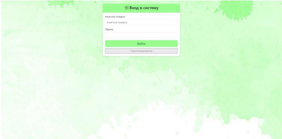
Рисунок 1 – Страница авторизации
