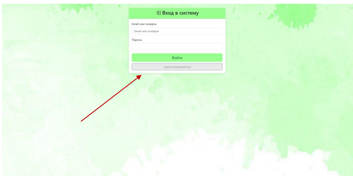
Рисунок 2 – Кнопка «Зарегистрироваться»
