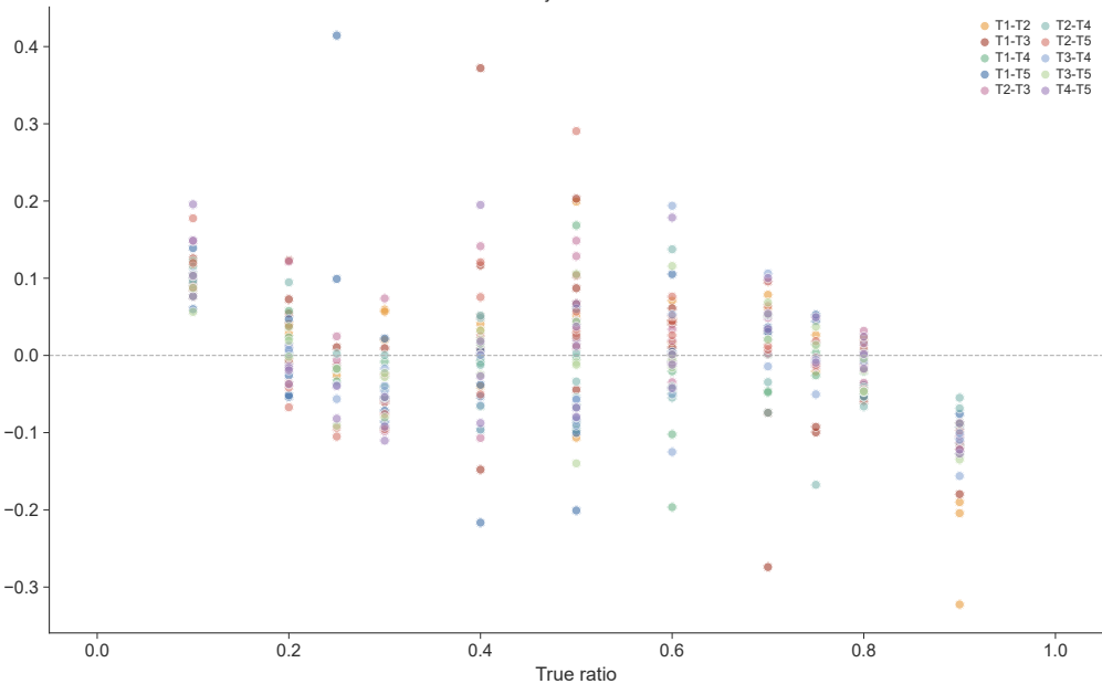
CARL-Proj + SVR residuals
